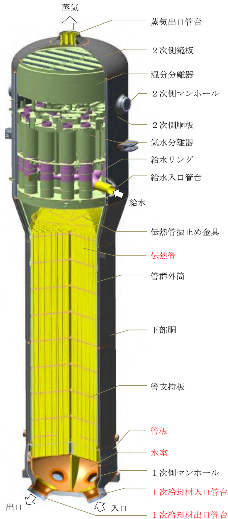
54F II 型 蒸気発生器
