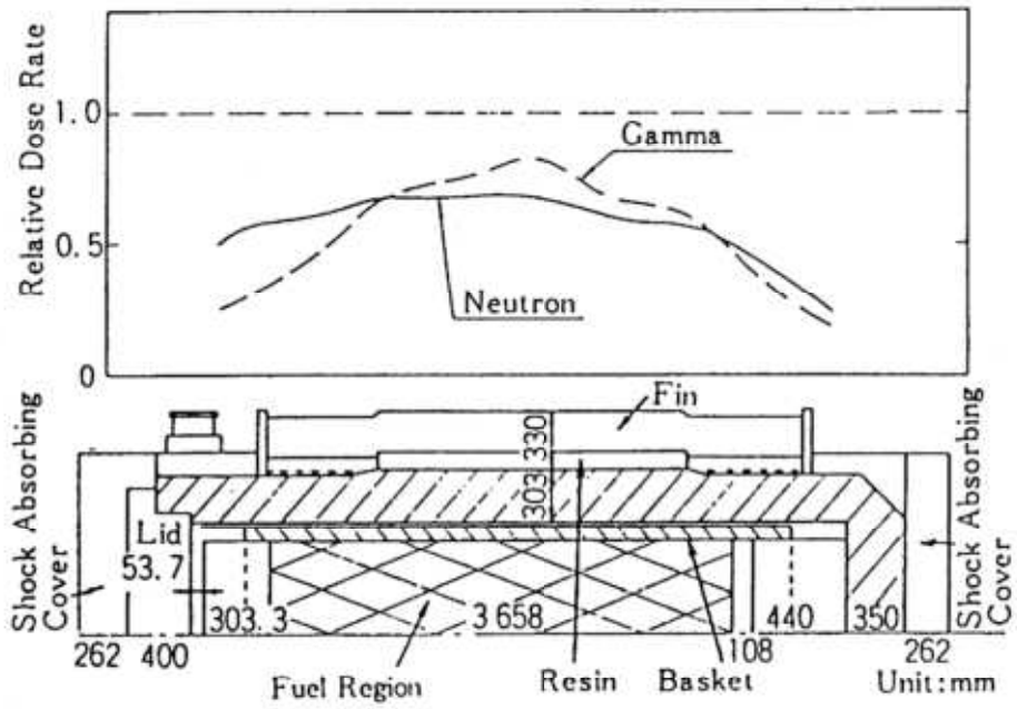
第12図 (1/2) DOT3.5の検証例 (その1) (23)
