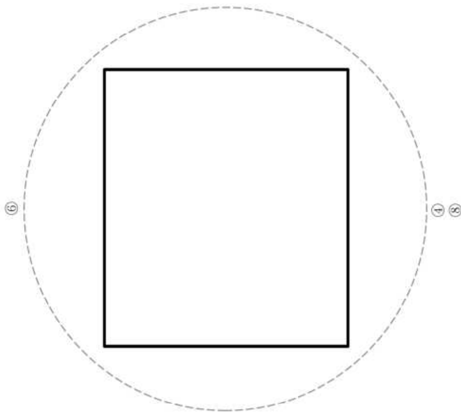
(注) ④, ⑥, ⑧の評価点位置は各方向での最大線量当量率となる位置を示している。 別紙5-1図(2/2) 特定兼用キヤスタクの表面から1 m離れた位置における代表評価点(水平断面)
