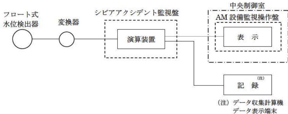
第3図 使用済燃料ピット水位（可搬型）の概略構成図
