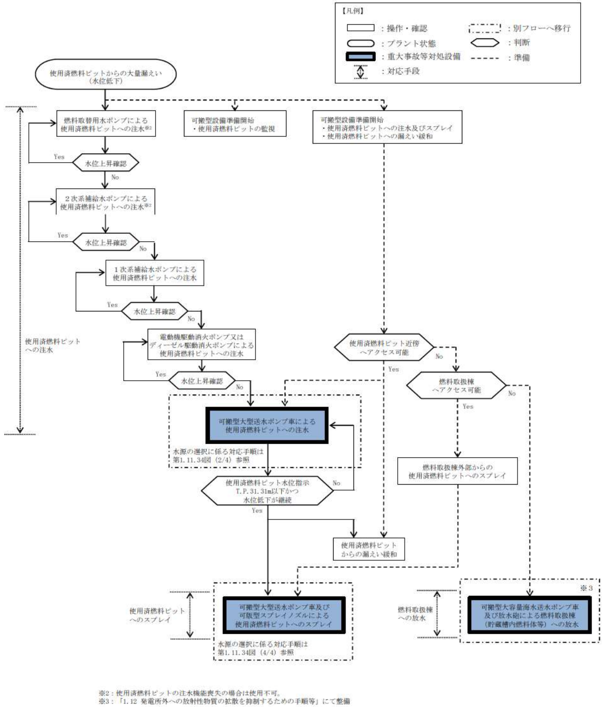
第 1.11.34 図 重大事故等時の対応手段選択フローチャート (3/4)
