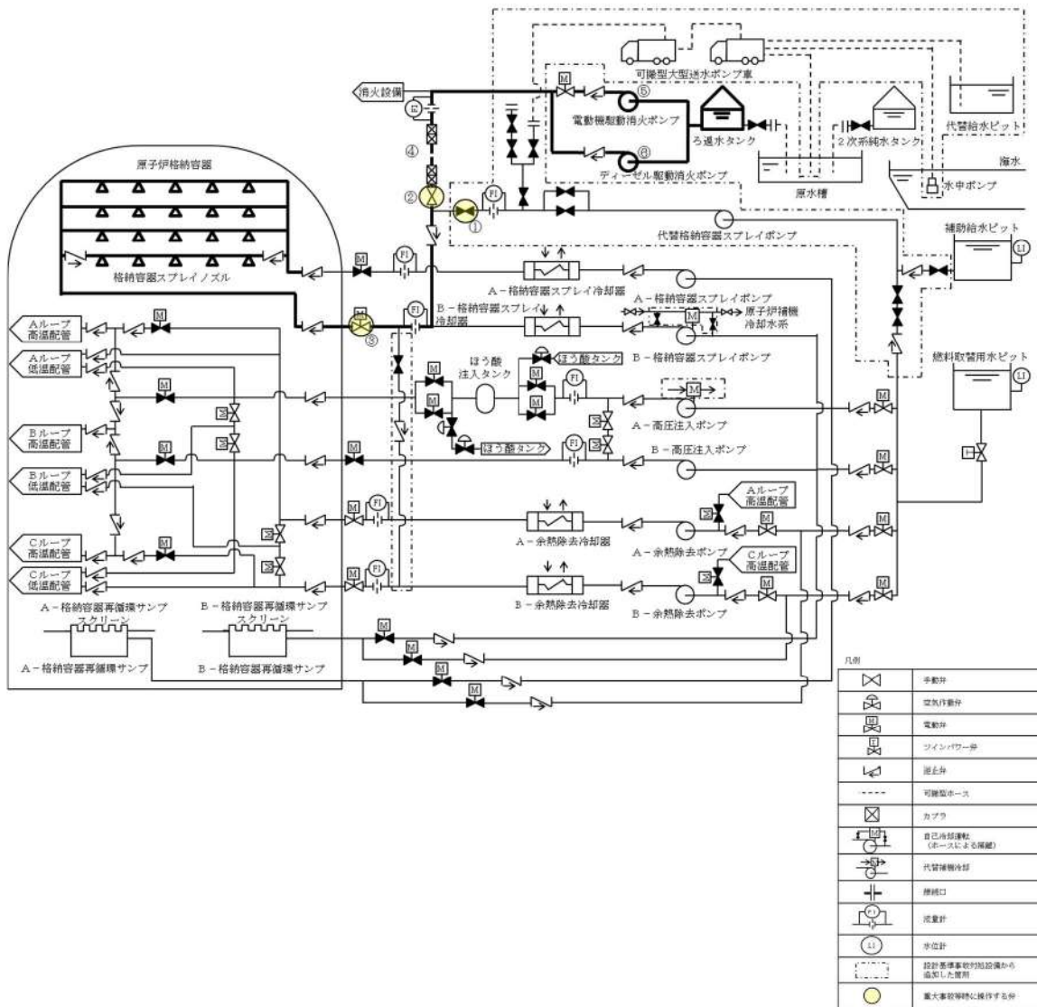
図 49-10-1 電動機駆動消火ポンプ又はディーゼル駆動消火ポンプによる原子炉格納容器内へのスプレイの概要図
