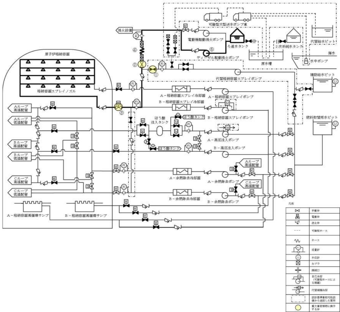
図 49-10-6 ディーゼル駆動消火ポンプによる原子炉格納容器内へのスプレイの概要図
