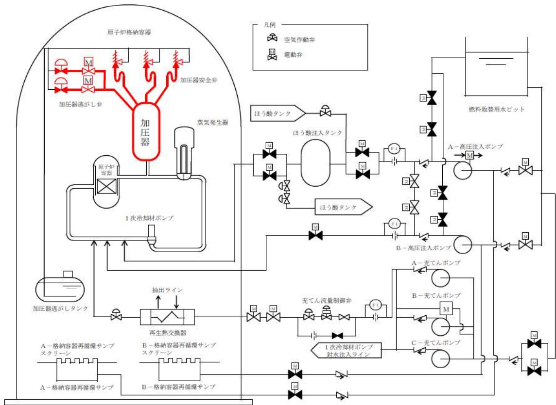
第 8 - 2 図 原子炉出力抑制 (手動) システム概要図
