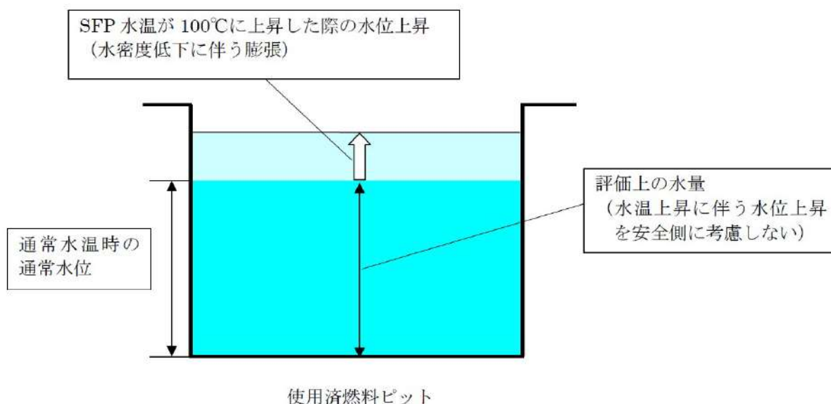
図1 使用済燃料ピットの水密度の概要
