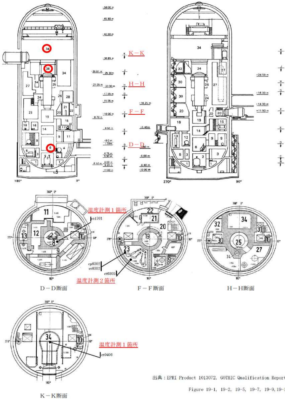
図 2 HDR 試験設備の概要
