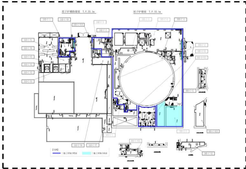
図1 溢水防護対策施工対象の壁及び床の配置図 (2/11)
