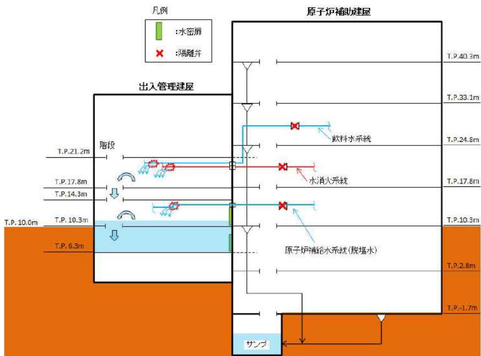
図 11-1 出入管理建屋の溢水概念図
