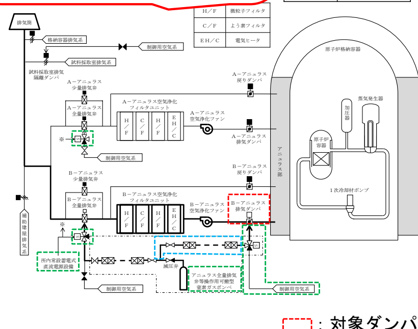
第1.16.14図 アニュラス空気浄化設備の運転
