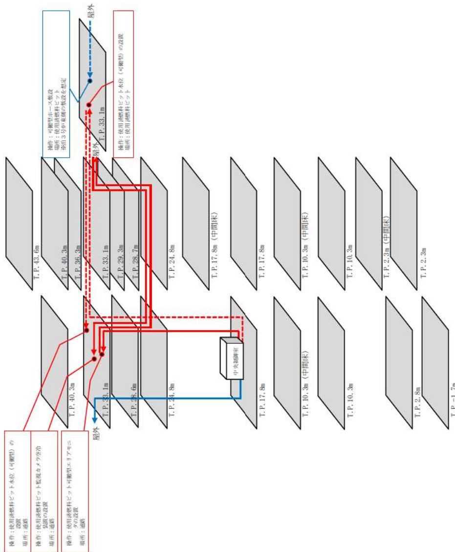
原子炉建屋 (周辺補機棟 (E/B) ) 原子炉建屋 (燃料取扱棟 (F/B/B) )
