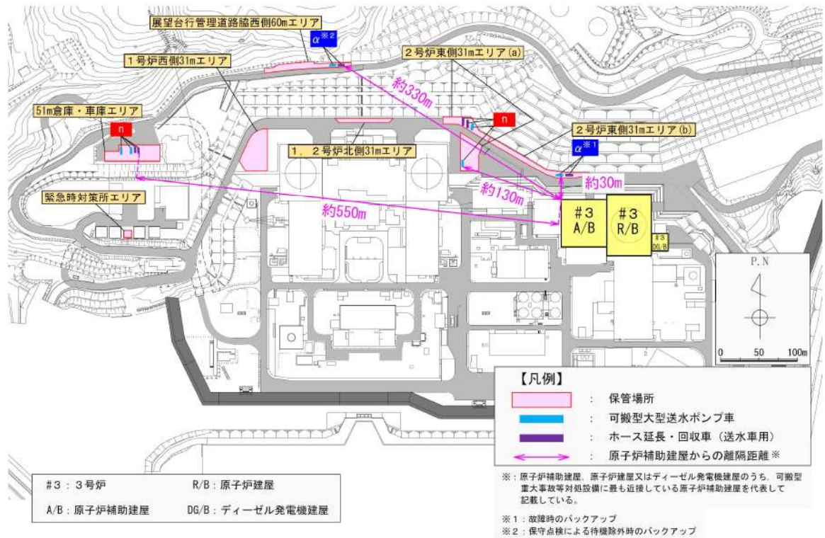
可搬型大型送水ポンプ車及びホース延長・回収車（送水車用）と原子炉補助建屋との離隔距離
