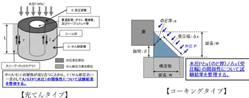
図 10 シリコンシーラント及び充てんシール材の耐水圧試験概要図
