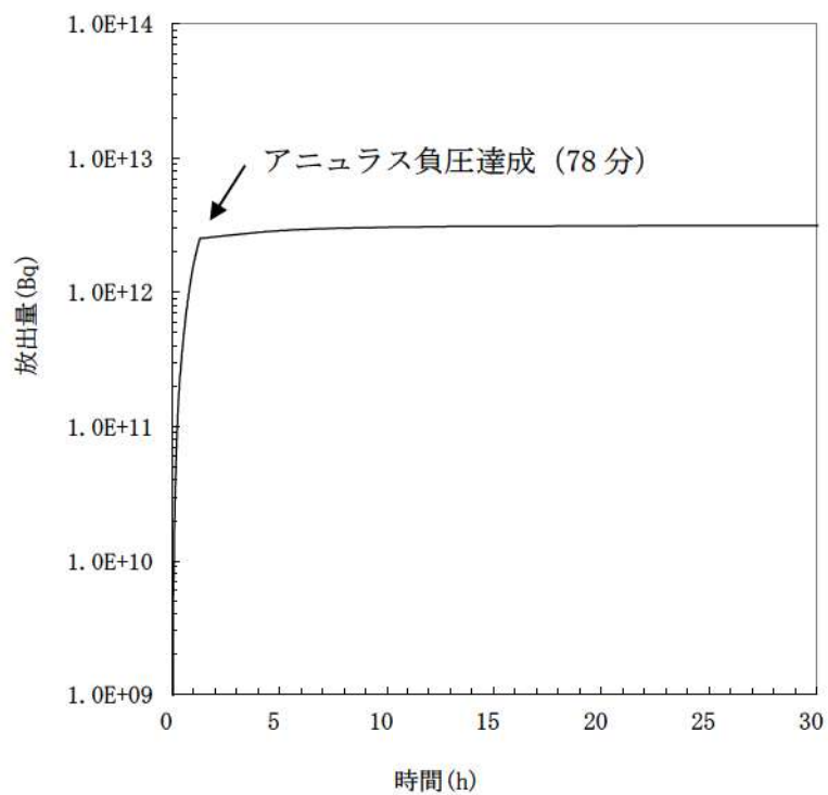
第2-5-13図 セシウム積算放出放射能量(GROSS値)の推移 (30時間)
