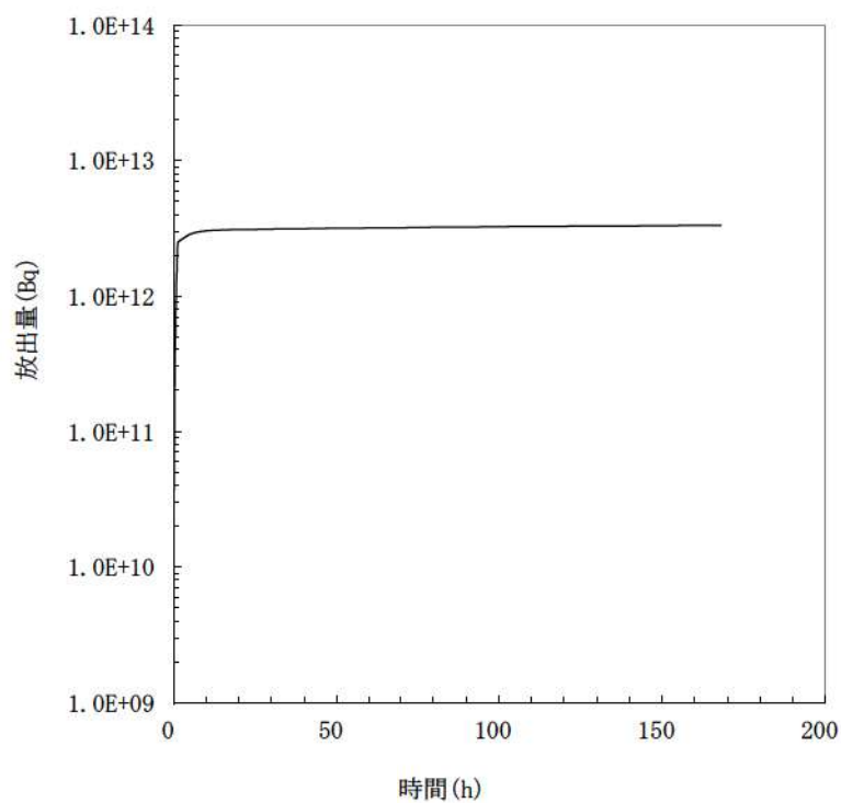
第 2-5-12 図 セシウム積算放出放射能量(GROSS 値)の推移 (7日間(168時間))
