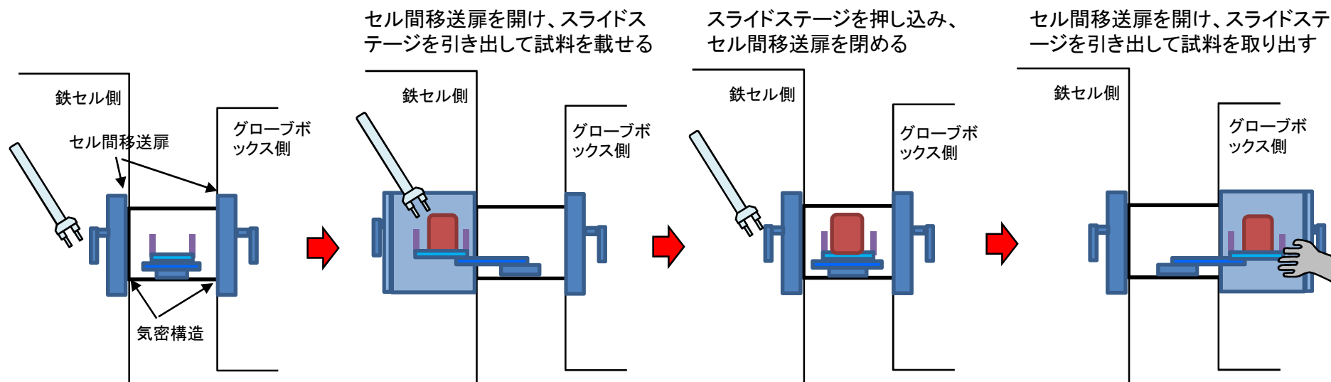
鉄セル、グローブボックス間の試料の移送方法
