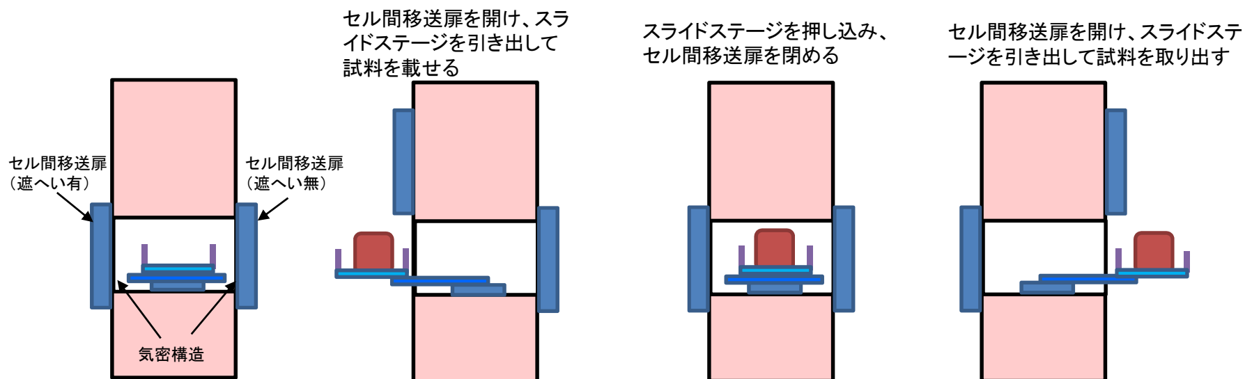
コンクリートセル、鉄セル間の試料の移送方法
