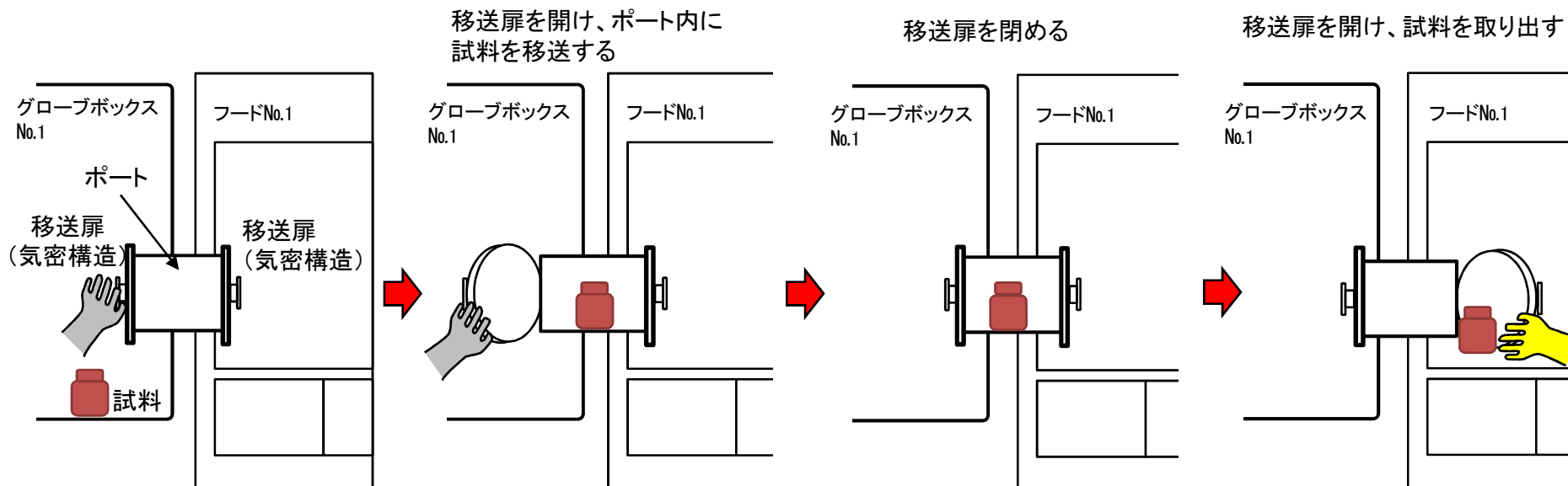
グローブボックスNo.1、フードNo.1間の試料の移送方法
