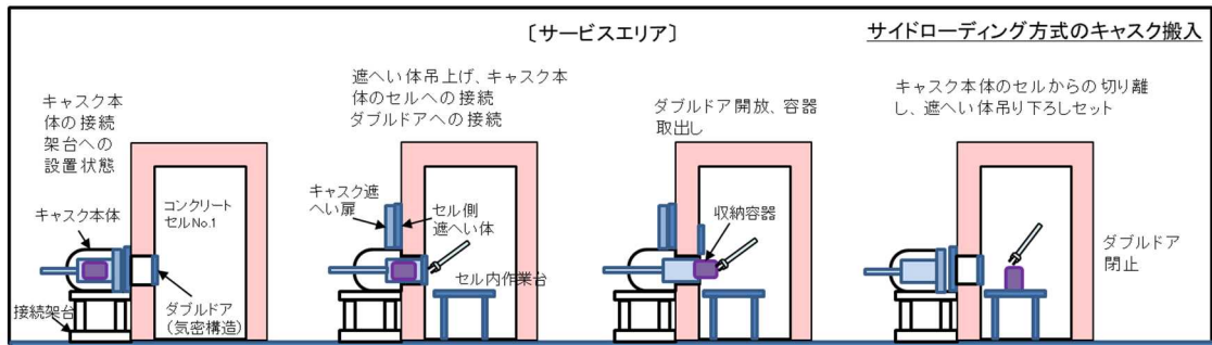
図 5.1.1-8 コンクリートセル No1 への搬入
