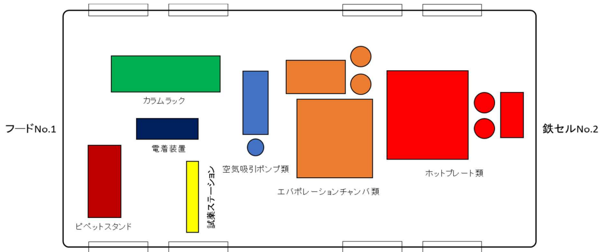
図 5.1.1-22 グローブボックス No. 1 の分析・試験装置等の配置イメージ
