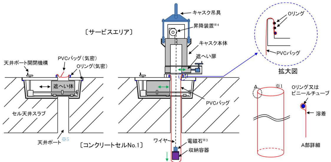
図 5.1.1-8 コンクリートセル No1 への搬入
