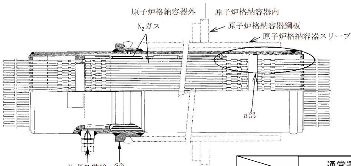
構造図
