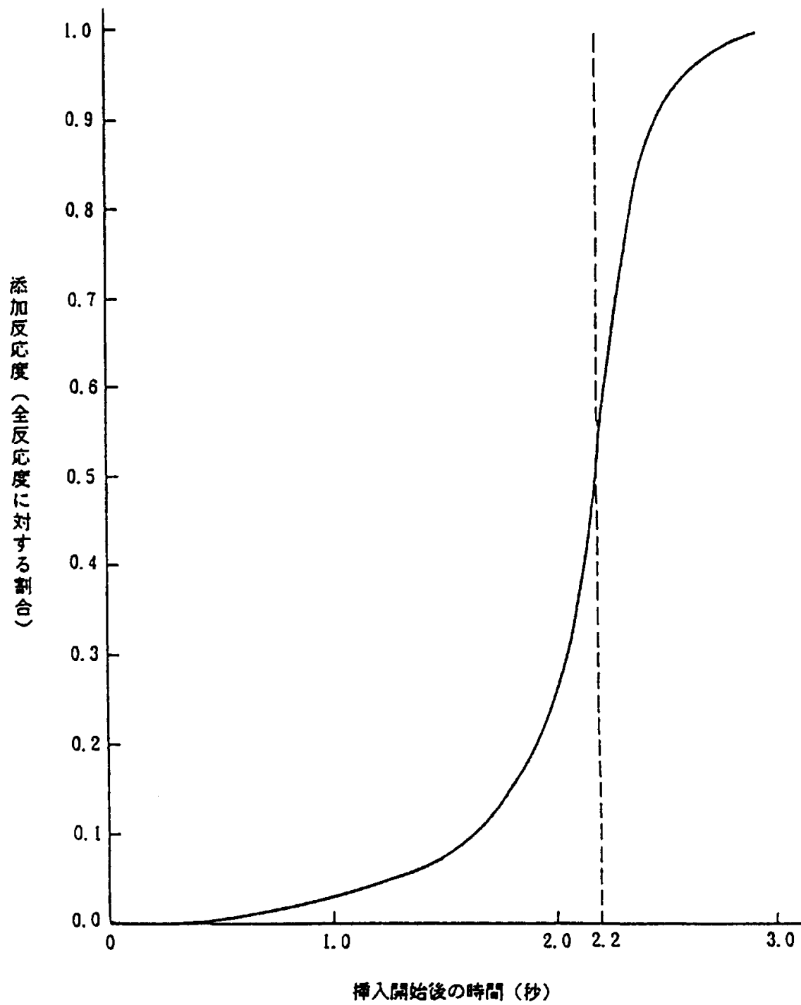
第 10.2 図 トリップ時の制御棒クラスタ挿入による反応度添加曲線
