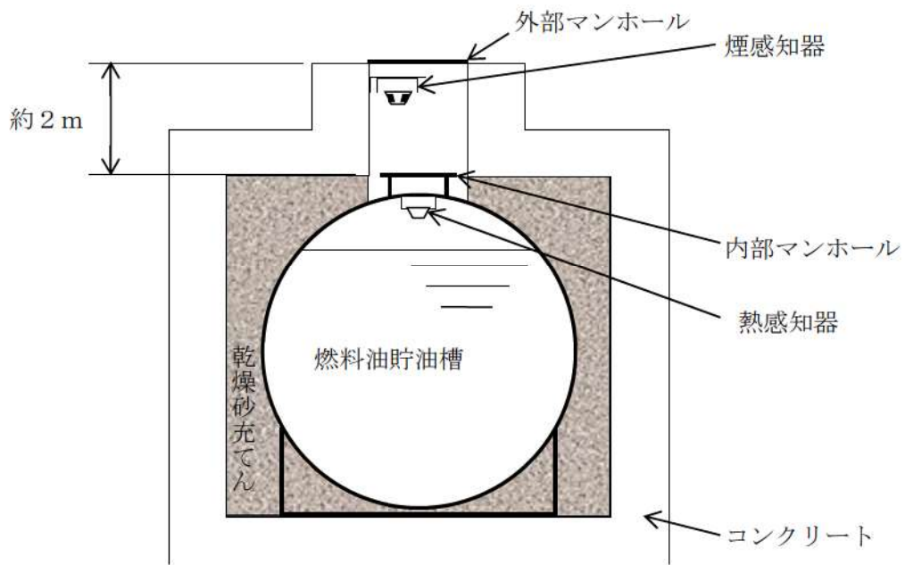
第 41-4-1 図 ディーゼル発電機燃料油貯油槽の火災感知器設置概要図
