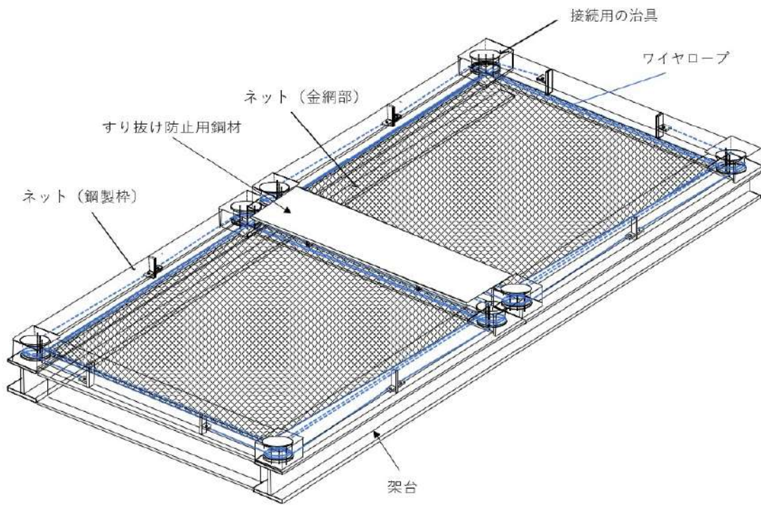
蛇巻防護ネットの構造イメージ
