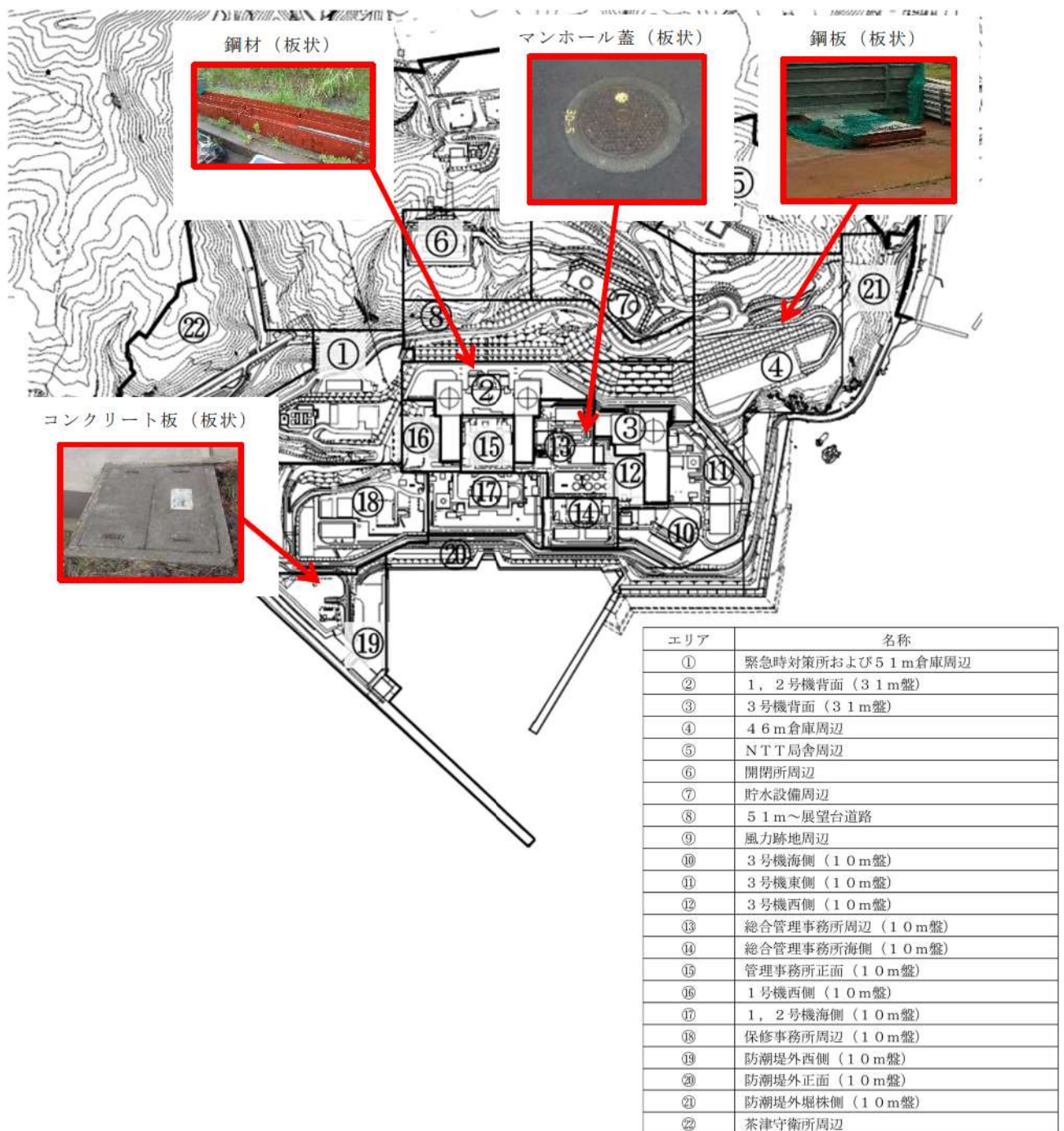
第 3.3.3 図 代表飛来物 (板状)
