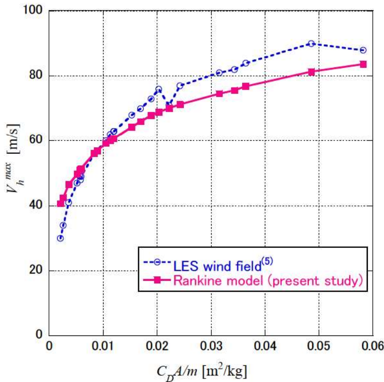
図3 空力パラメータと飛来物速度の関係
