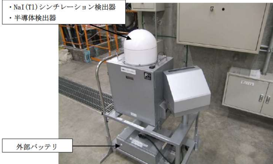
(可搬型モニタリングポストの写真)
