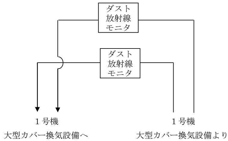
図 2. 15-1 1号機 ダスト放射線モニタ検出器 系統概略図 (大型カバー換気設備出口)
