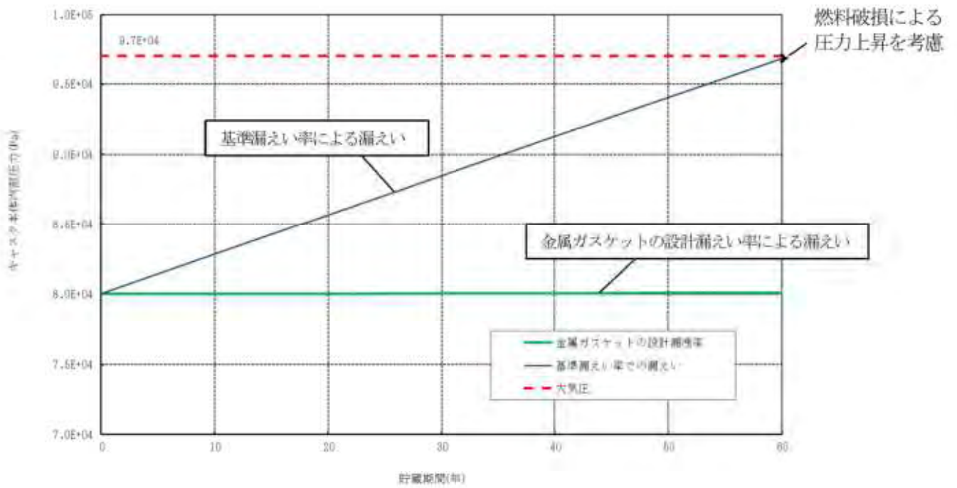
第5図 特定兼用キャスク内部圧力の経時変化
