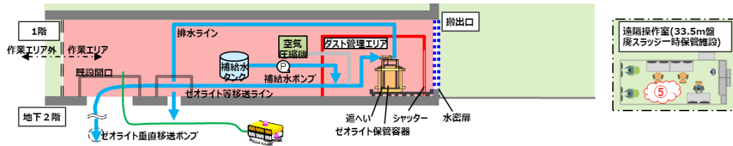
図 2.12.2-4 地上階での作業状況 (4/8)
