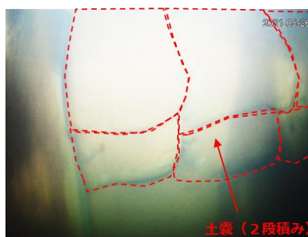
② 最下階の様子 (HTI) (水中)
