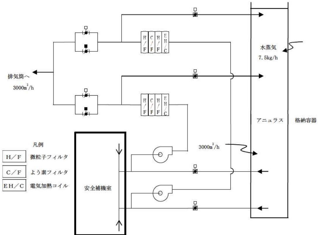
第2図 泊3号炉 アンユラス空気浄化設備系統構成
