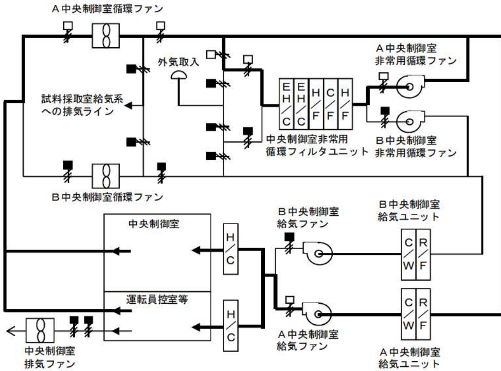
第3図 中央制御室空調装置の概要図
