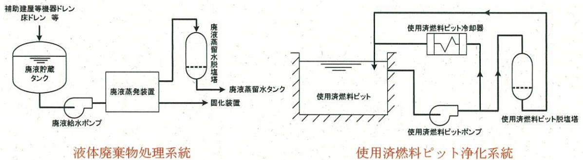
図1. 脱塩塔が設置されている系統（概略図）
