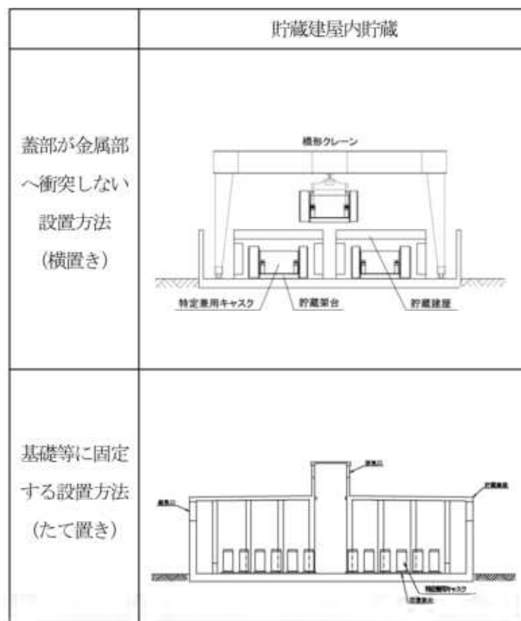
第12図 特定兼用キャスク貯蔵施設概要図 (例)
