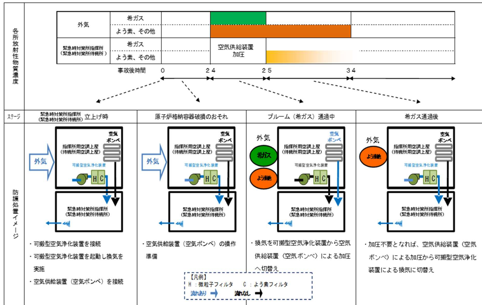
図10 ブルーム通過時の換気設備の運用<<換気空調設備等の運用イメージ>>
