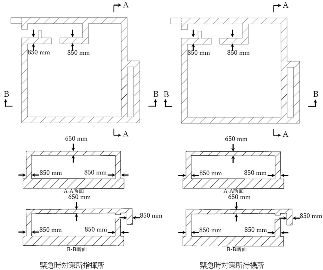
図9 緊急時対策所 遮蔽説明図
