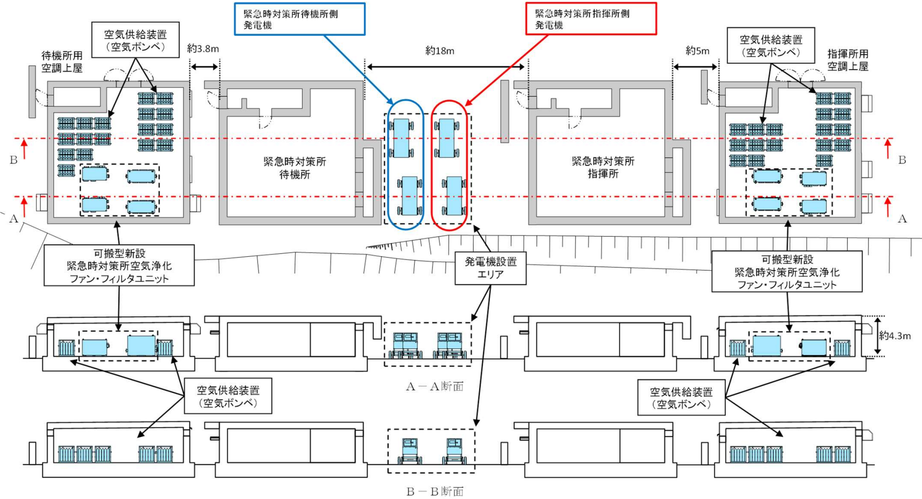
図2 緊急時対策所 周辺図
