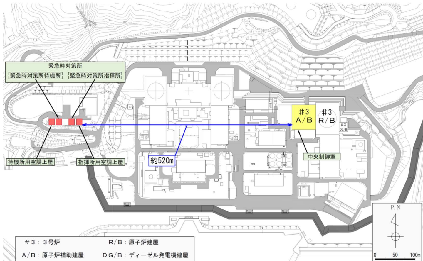
図7 緊急時対策所配置図
