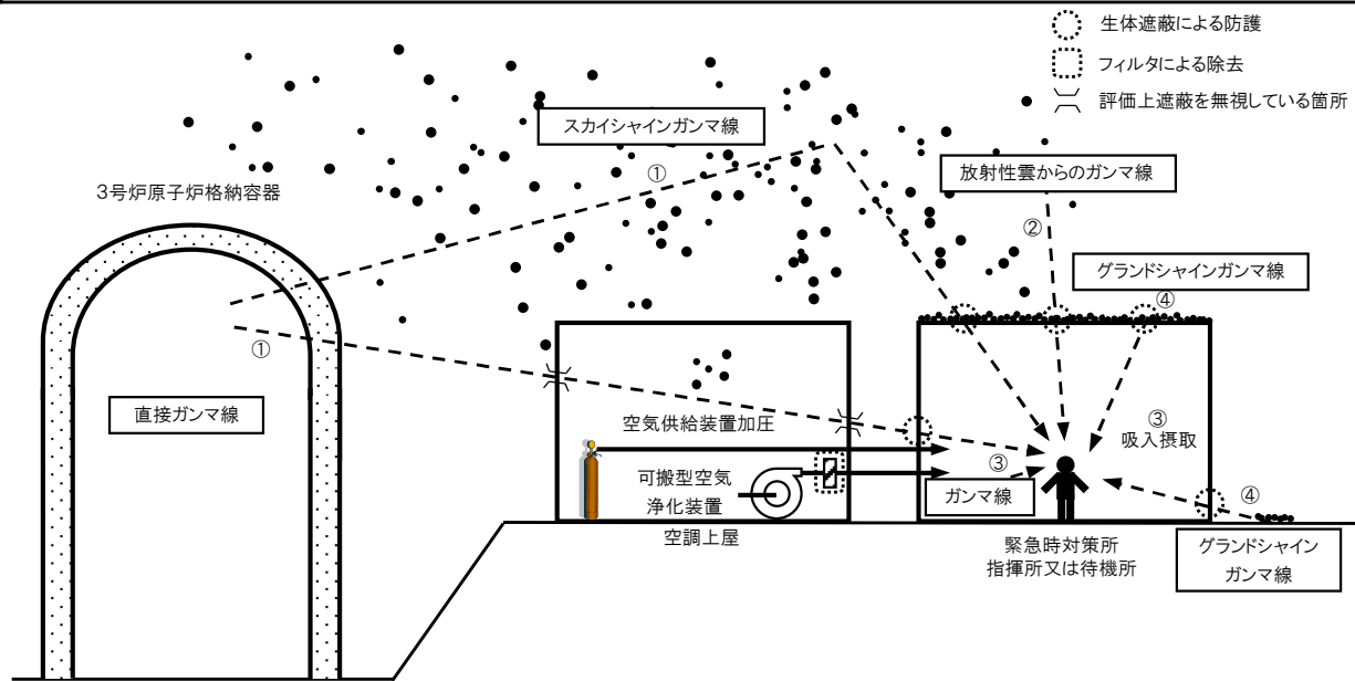
図14 緊急時対策所の居住性に係る経路イメージ図
