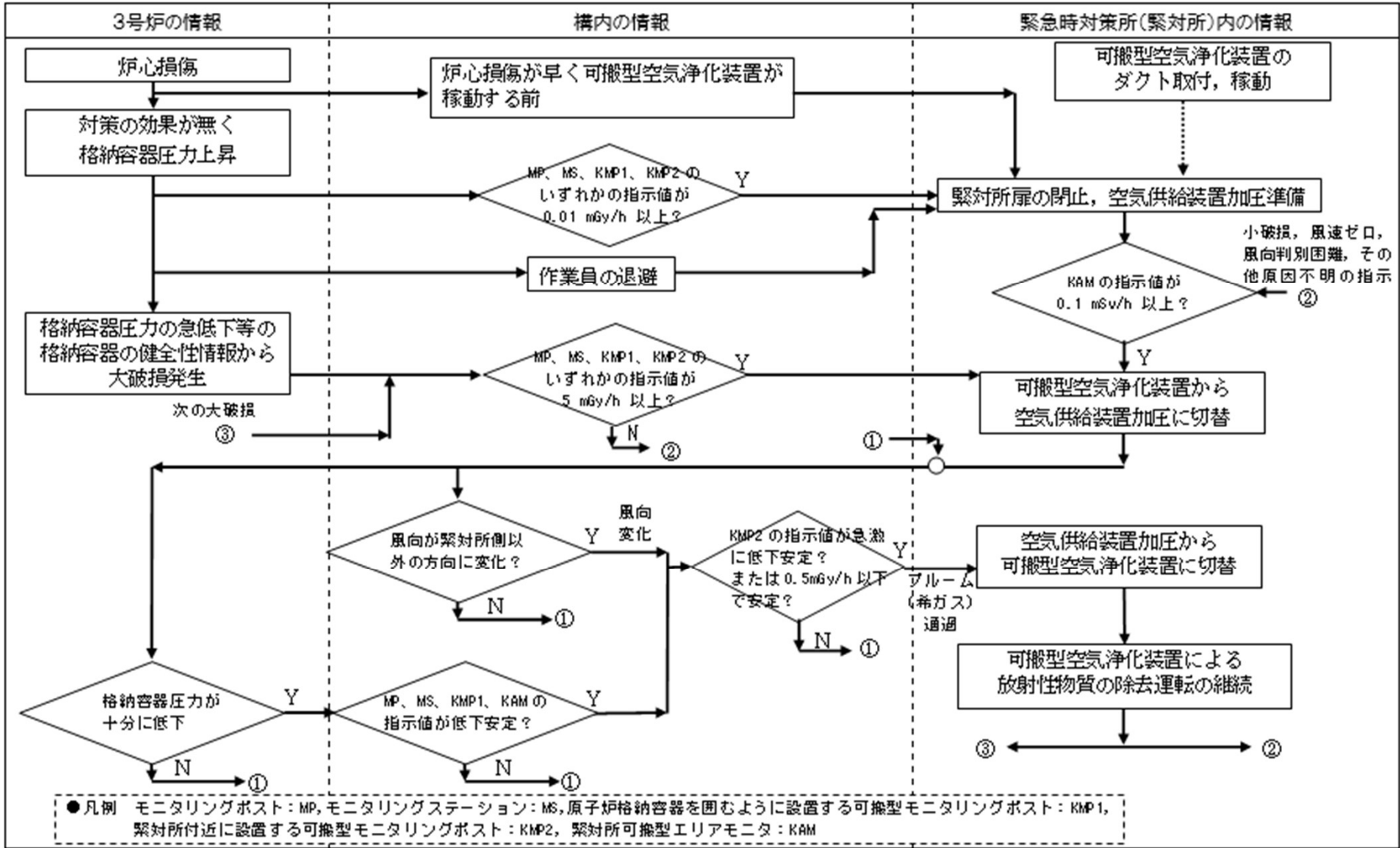
図15 緊急時対策所換気空調設備の運用基本フロー
