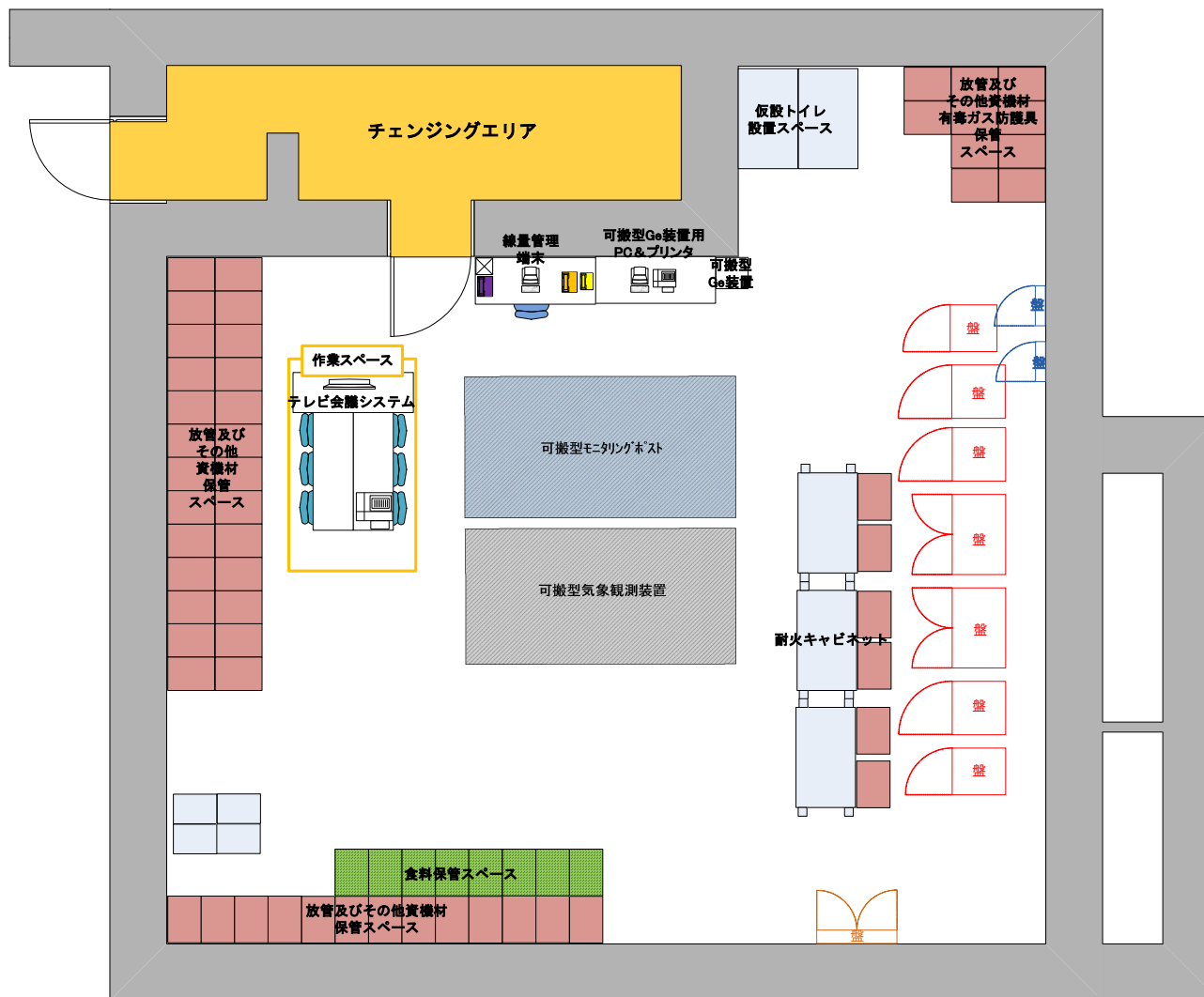
図4 緊急時対策所待機所レイアウトイメージ図
