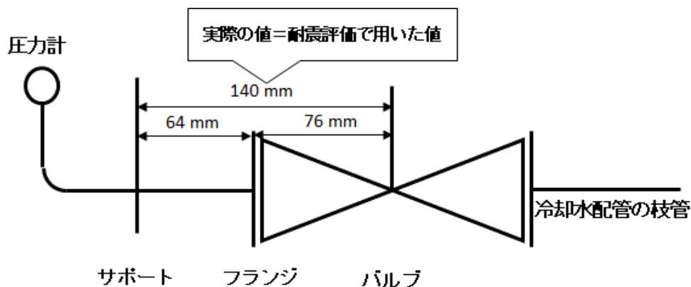
図 冷却水配管の枝管の概略
