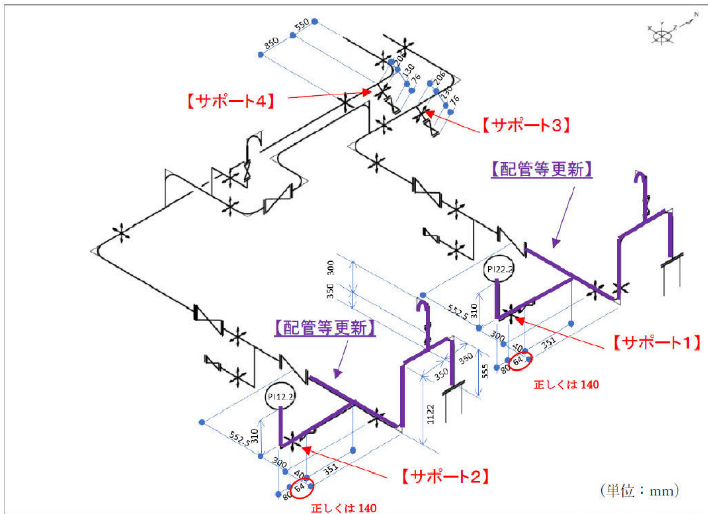
別図-2 サポートの設置位置及び配管の一部更新範囲 (廃止措置計画変更認可申請書抜粋)
