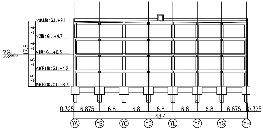
図-7 A-A断面図 (単位:m)
