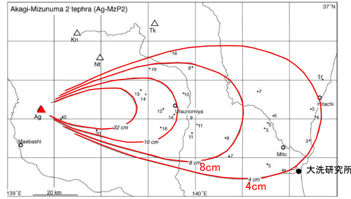
第20図 赤城水沼2テフラ(Ag-MzP2)の分布 数字は降下火砕堆積物の層厚で、単位はcm。Ag = 赤城火山；Hu = 燧ヶ岳火山；Kn = 鬼怒沼火山；Ni = 男体火山；Tk = 高原火山。
