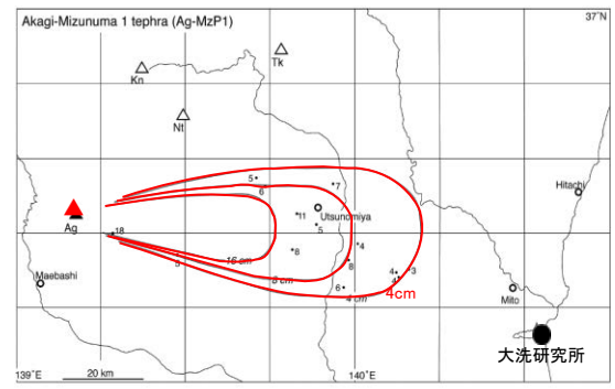
第19図 赤城水沼1テフラ(Ag-MzP1)の分布 数字は降下火砕堆積物の層厚で、単位はcm。Ag = 赤城火山；Hu = 燧ヶ岳火山；Kn = 鬼怒沼火山；Ni = 男体火山；Tk = 高原火山。
