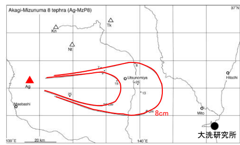
第22図 赤城水沼8テフラ(Ag-MzP8)の分布 赤城水沼8テフラの等層厚線図 (山元 (2013a) に加筆)
