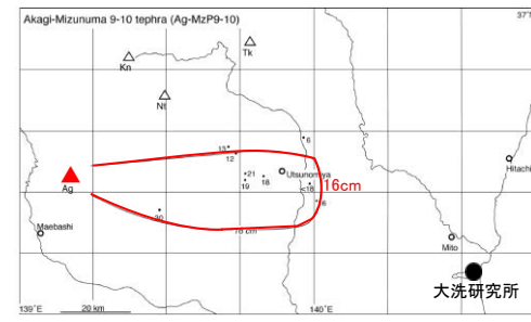
第23図 赤城水沼9-10テフラ(Ag-MzP9-10)の分布 赤城水沼9-10テフラの等層厚線図 (山元 (2013a) に加筆)
