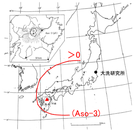
図 2.1-15 阿蘇3テフラ (Aso-3) と阿蘇3テフラ (Aso-3 (pf)) の分布と主な産出地点。●Aso-3 ▲Aso-3 (pf)。点線内は火砕流堆積物 (Aso-3 (pf)) の分布範囲を示す。左上の図は小野・渡辺(1985)に加筆。
