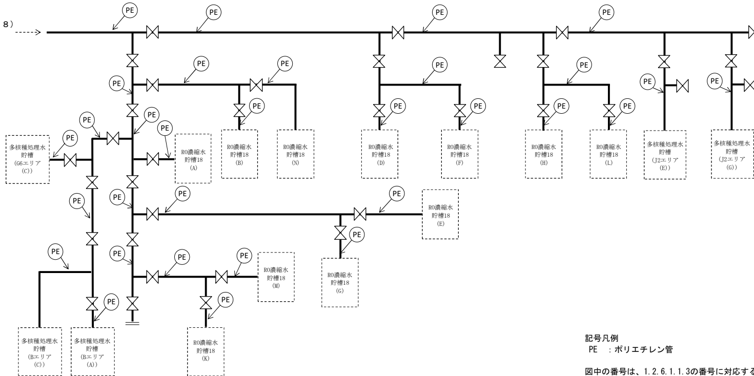
図-1 配管概略図 (14/18)
