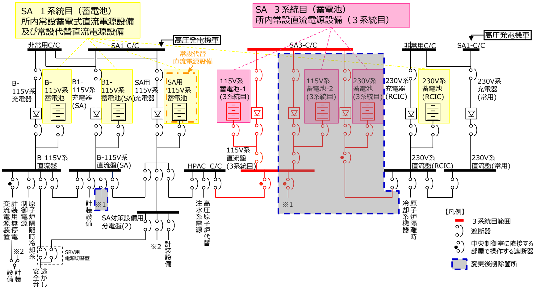
図1 所内常設直流電源設備（3系統目）概略系統図（補正時）
