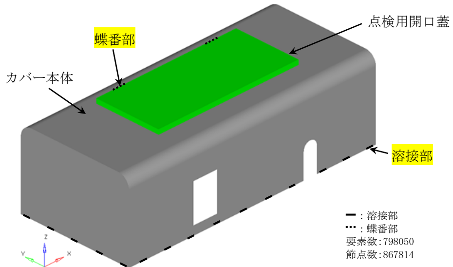
図 3-4 解析モデル
