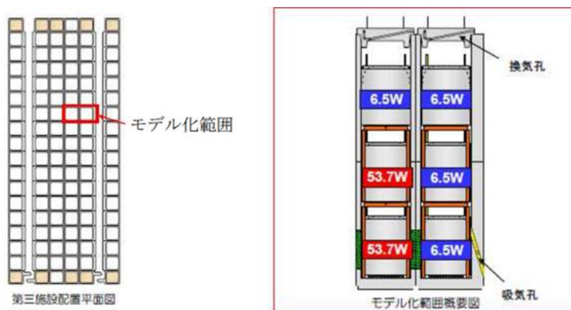
図 2.14.5-1 第三施設温度評価の評価体系概念
