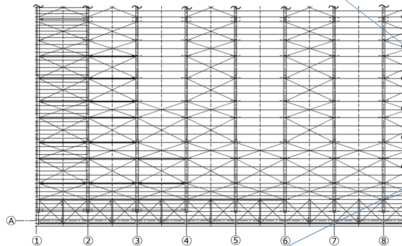
屋根架構
