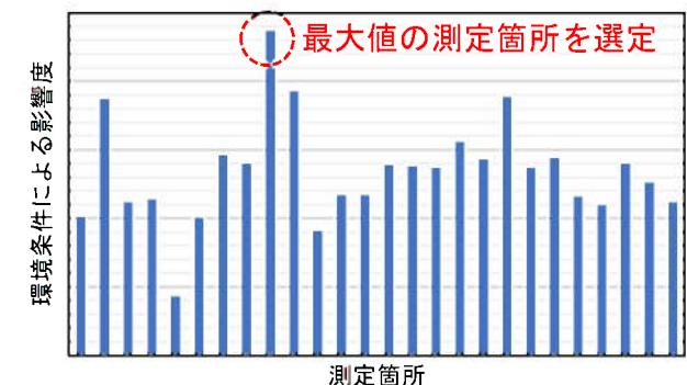
環境条件による影響度の確認結果の事例 (川内1号炉 原子炉補助建屋 内壁及び床)
