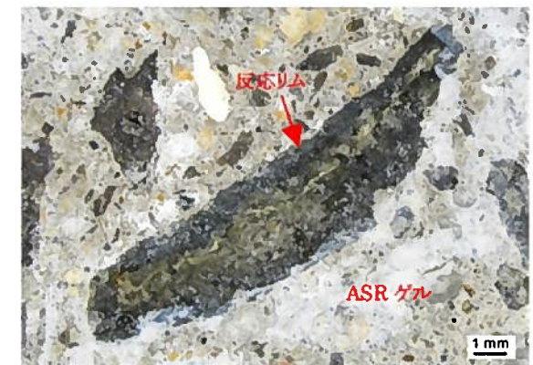
実体顕微鏡観察による観察写真の例 (川内1号炉 原子炉格納施設等 外部遮蔽壁)
