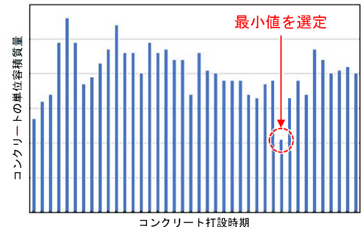
建設時のコンクリート単位容積質量の事例 (川内1号炉 原子炉格納施設等 外部遮蔽壁)
