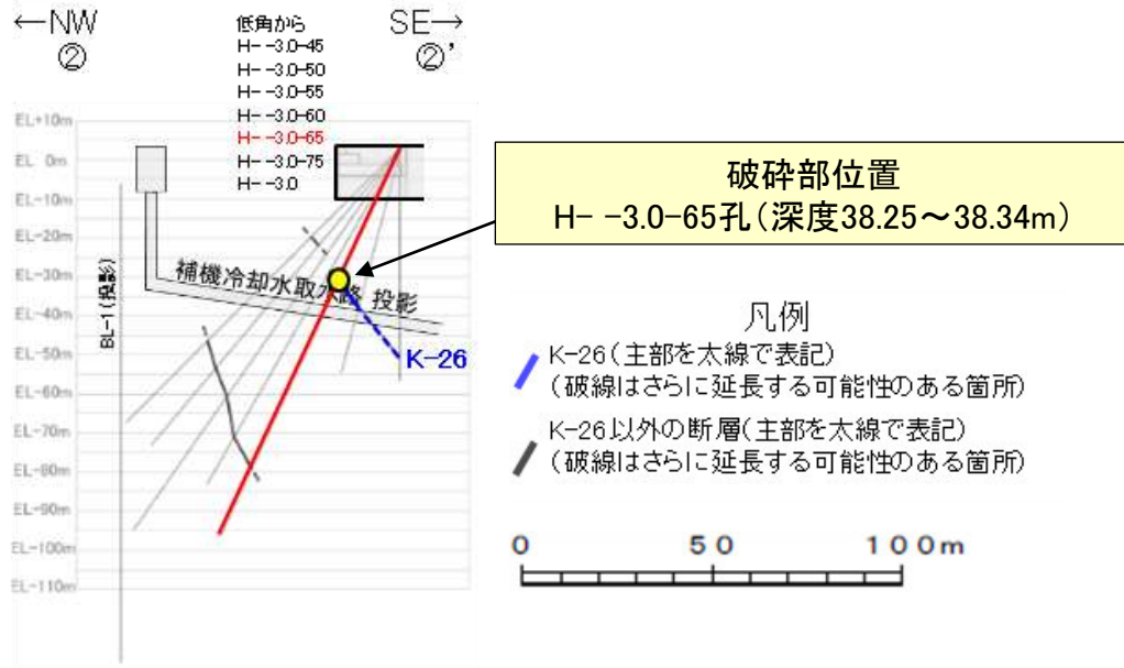
②-②' 断面図
