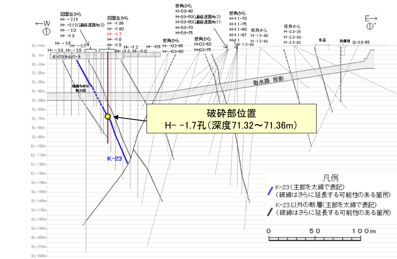
①-①'断面図
