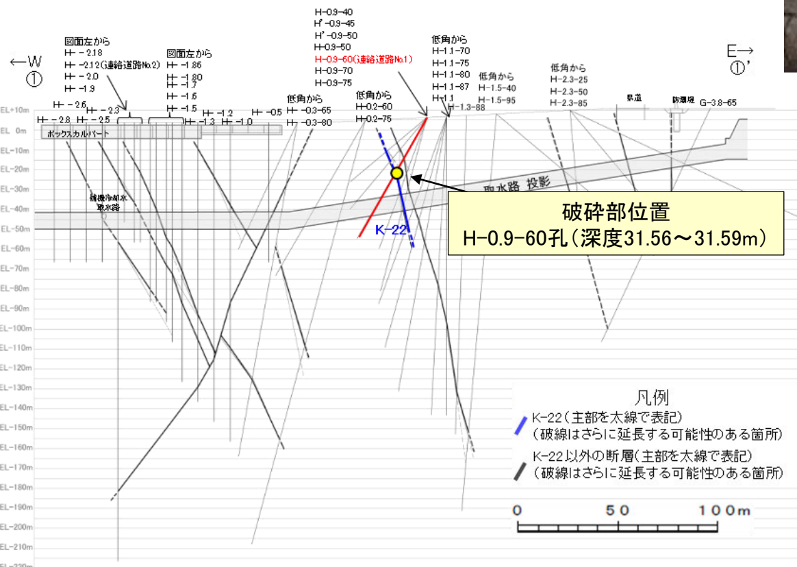
①-①'断面図
