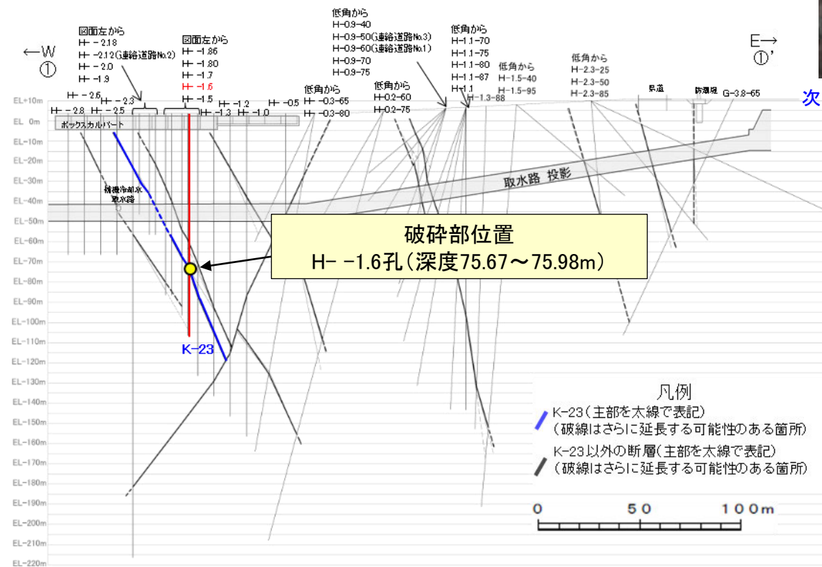
①-①'断面図
