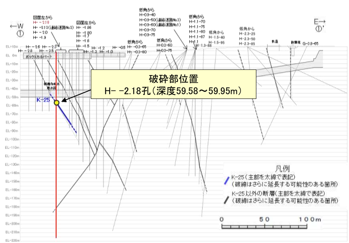
①-①'断面図
