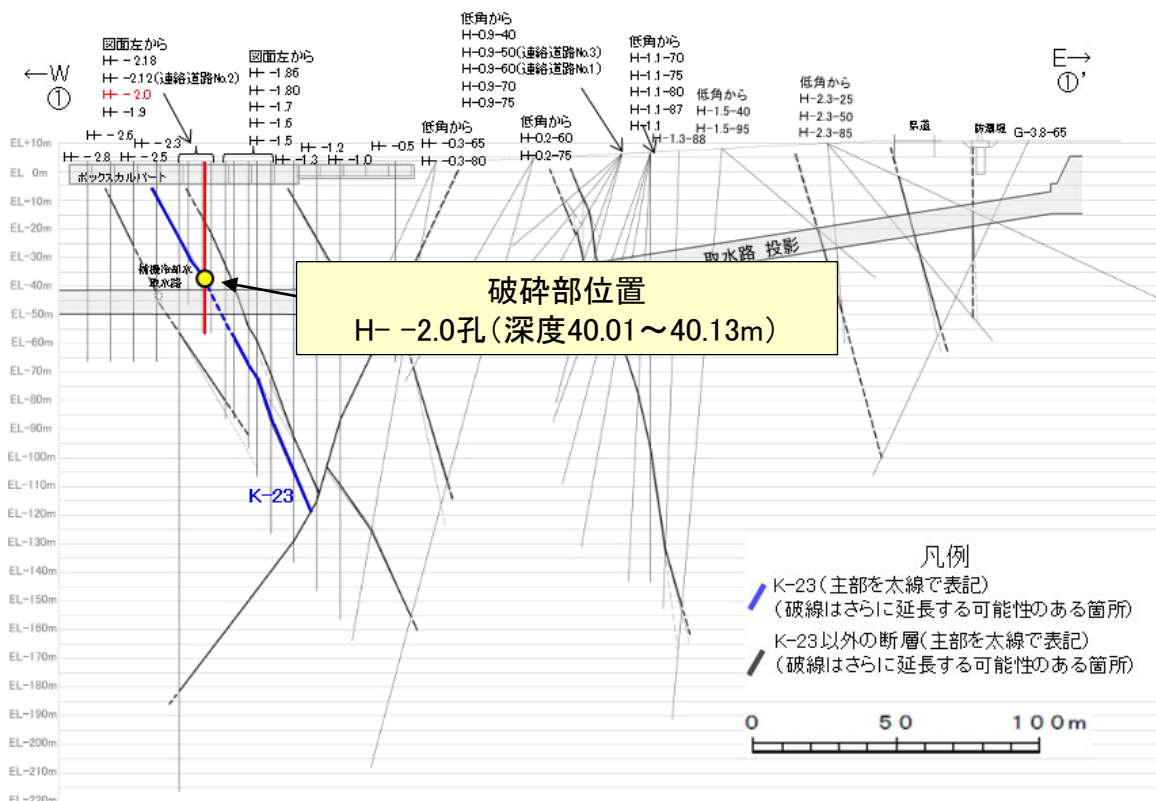
①-①' 断面図
