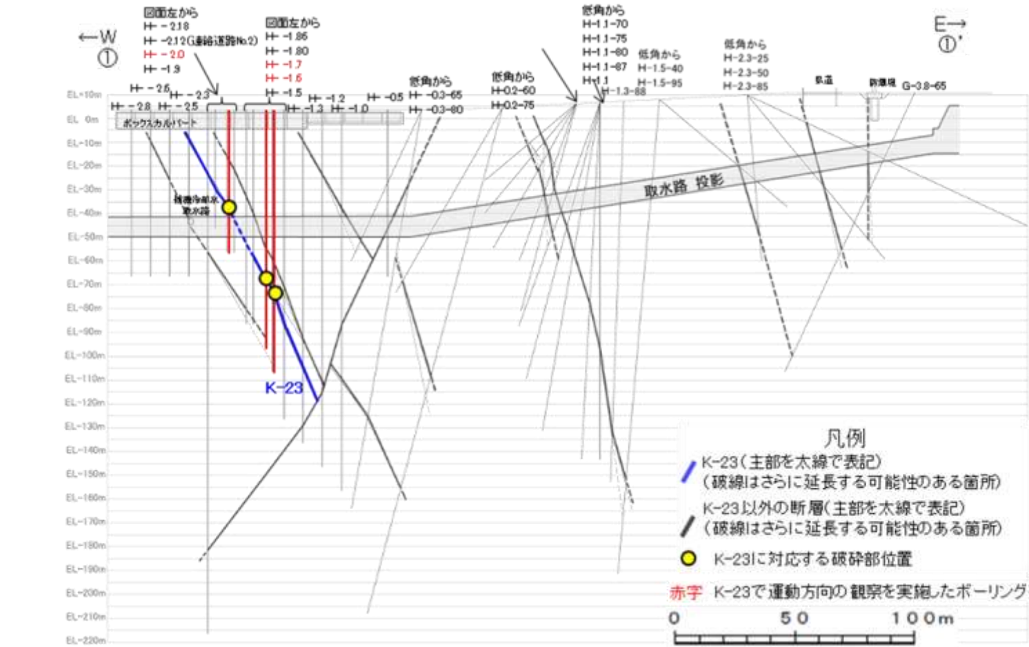
①-①' 断面図
