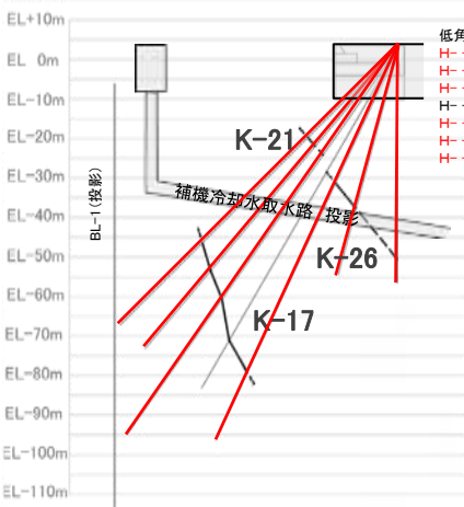
②-②' 断面図
