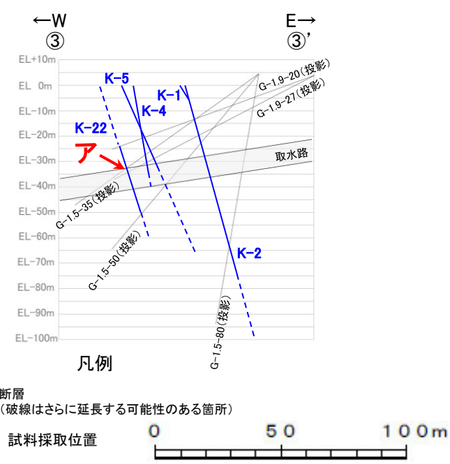
③-③' 断面図
