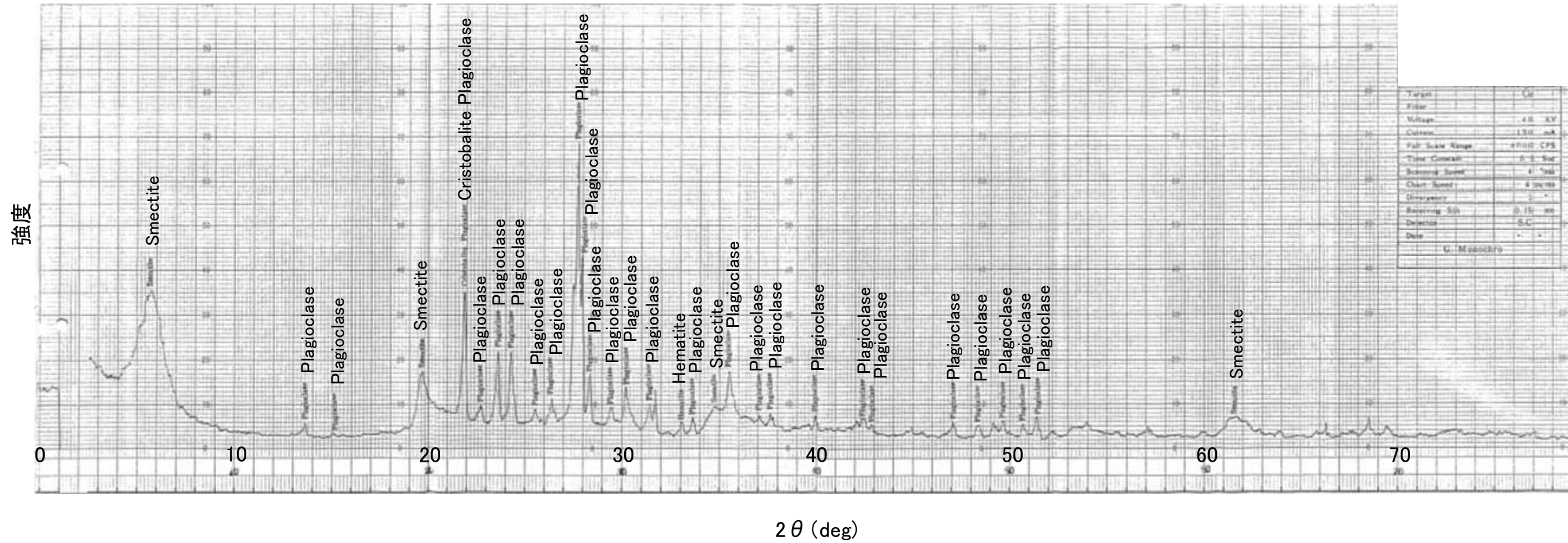
回折チャート
