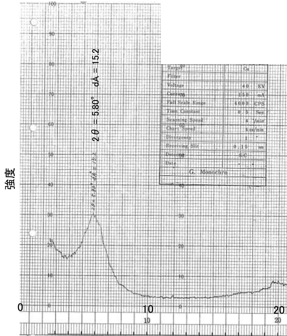
2θ (deg) 回折チャート
