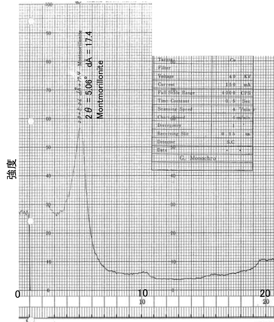
2θ (deg) 回折チャート (EG処理)
