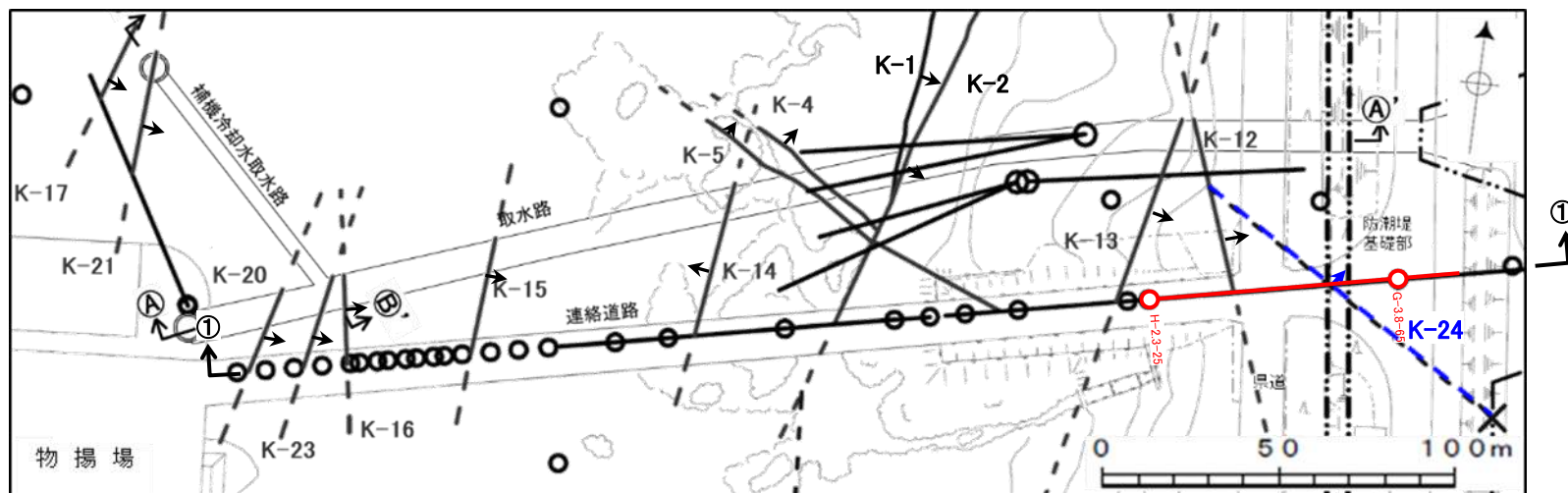
平面図
