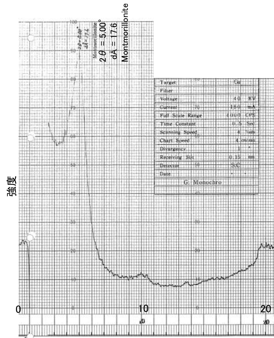
2θ (deg) 回折チャート (EG処理)
