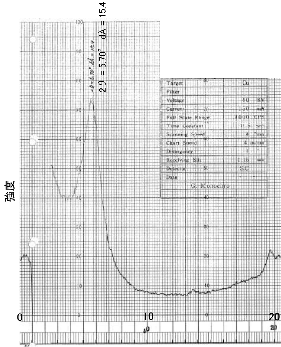
2θ (deg) 回折チャート
