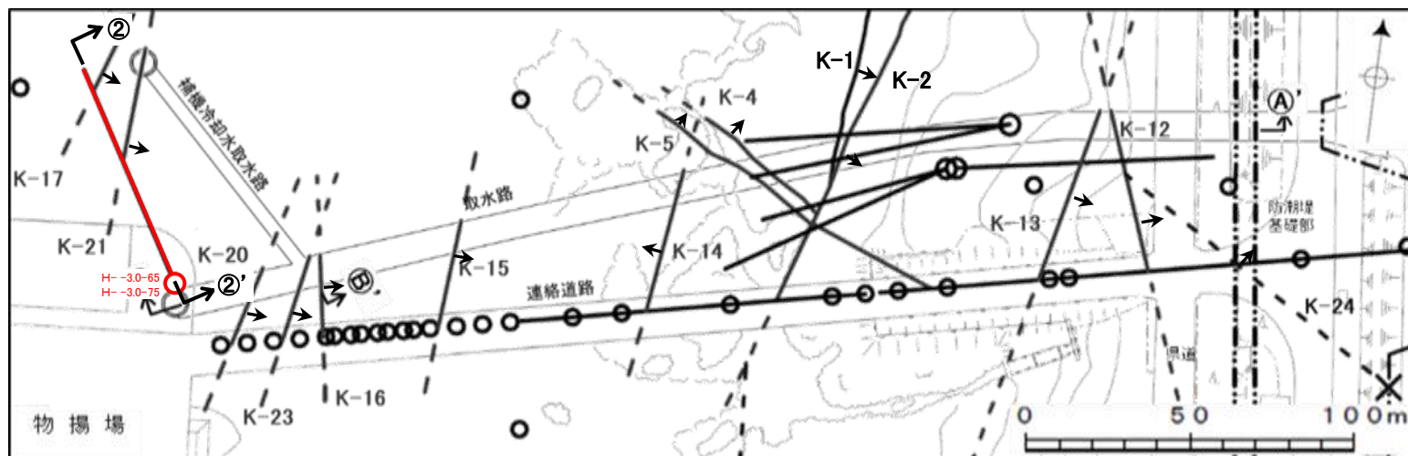
平面図
