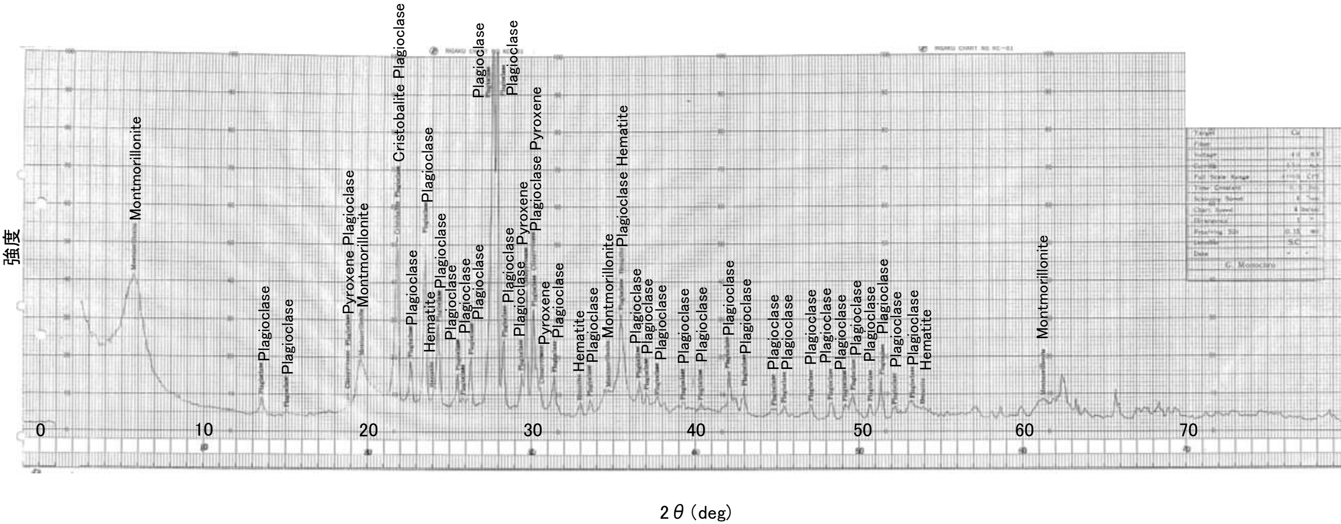
回折チャート
