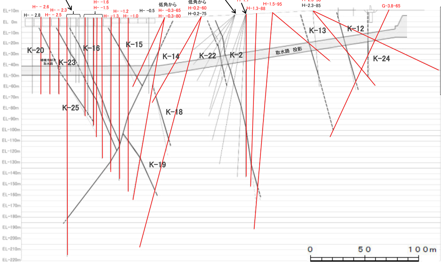
①-①' 断面図
