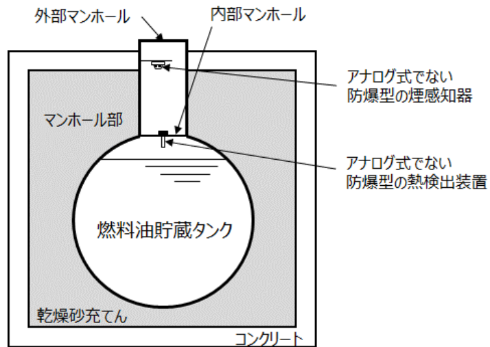
第 3-2-9 図 [ ] の火災感知器配置図（断面図）
