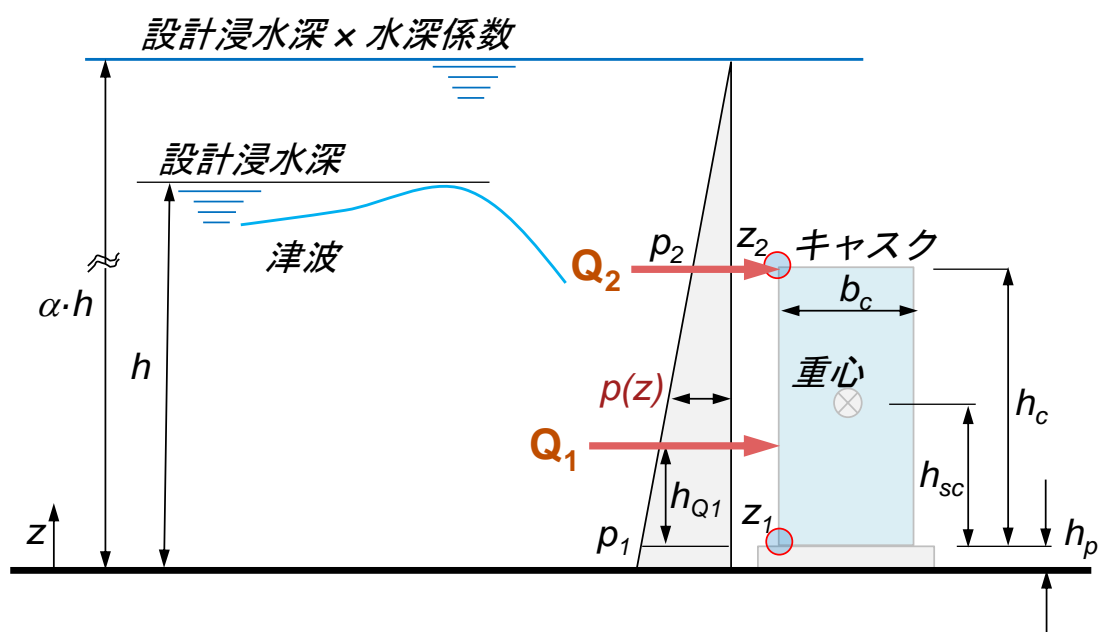
図 2 津波波力の作用形態
