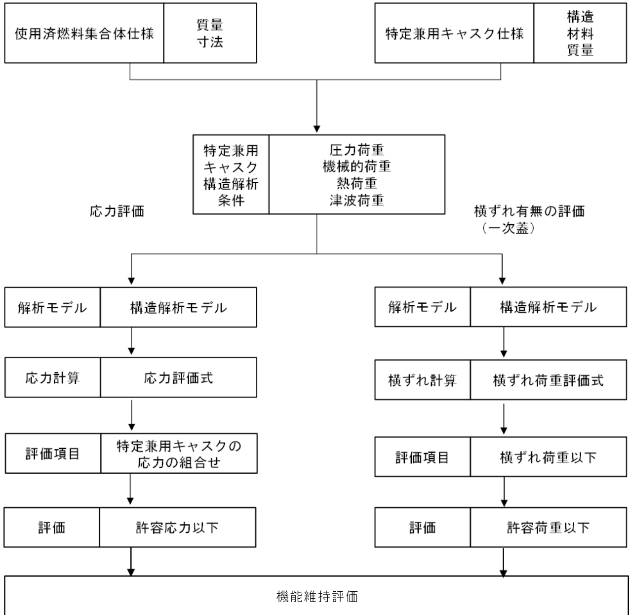
図1 津波荷重作用時の機能維持評価フロー
