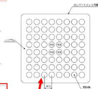
燃料集合体は空間の中央に配置
