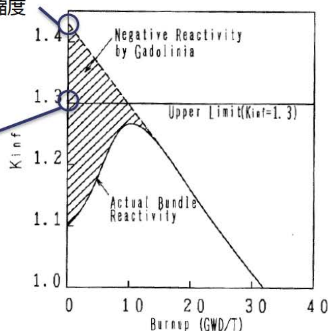
収納するBWR燃料の反応度特性の例[1]
