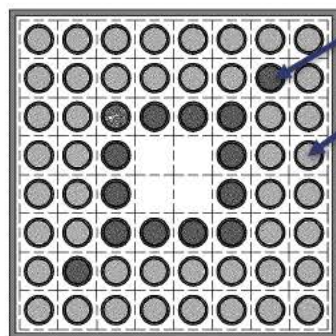
冠水状態の燃料モデル
