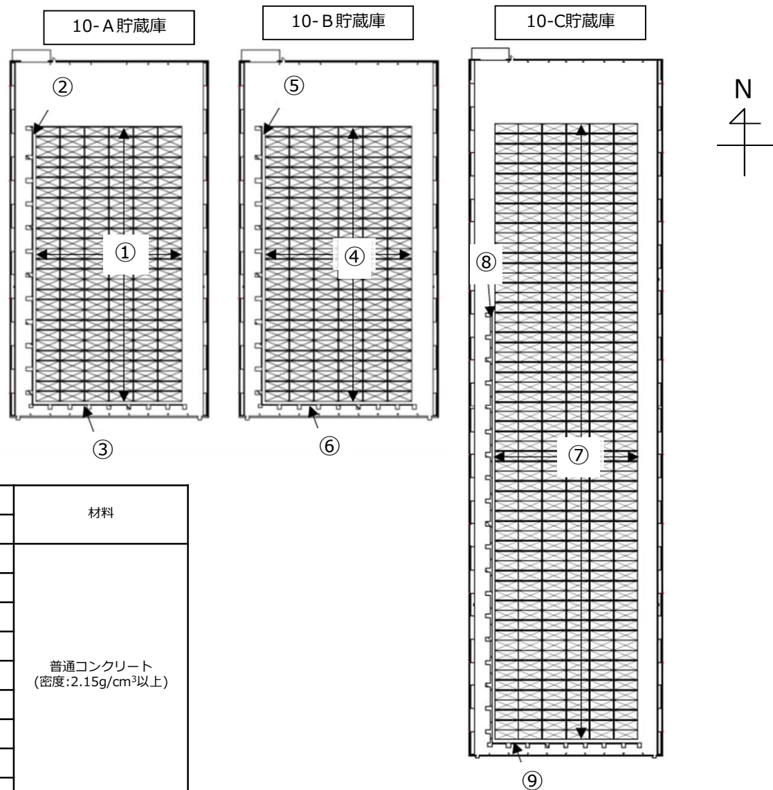
<固体廃棄物貯蔵庫第10棟の遮蔽に関する構造図>
