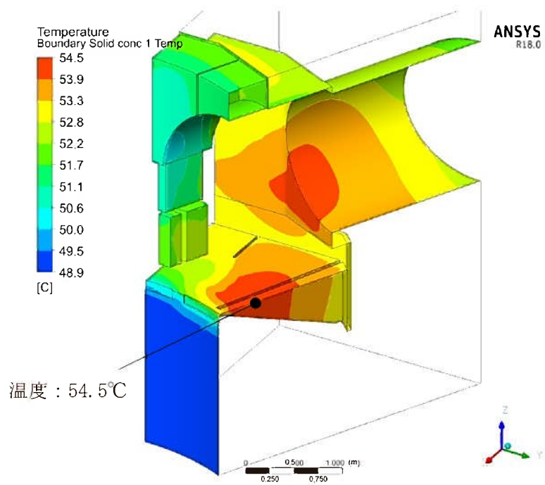
図7 原子炉容器サポート回りのコンクリートの温度分布
