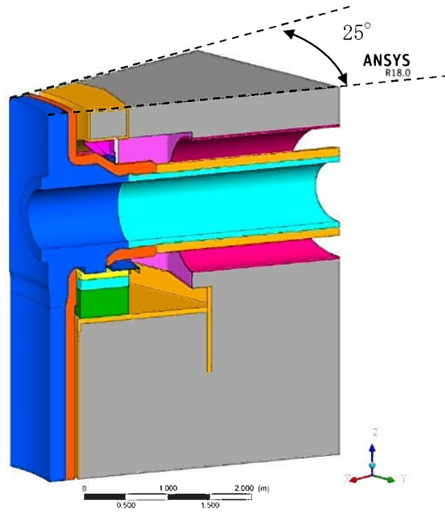
図5 解析モデル (全体)
