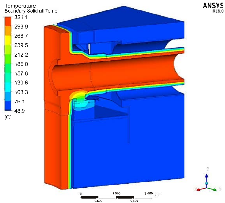
図6 解析モデル全体の温度分布
