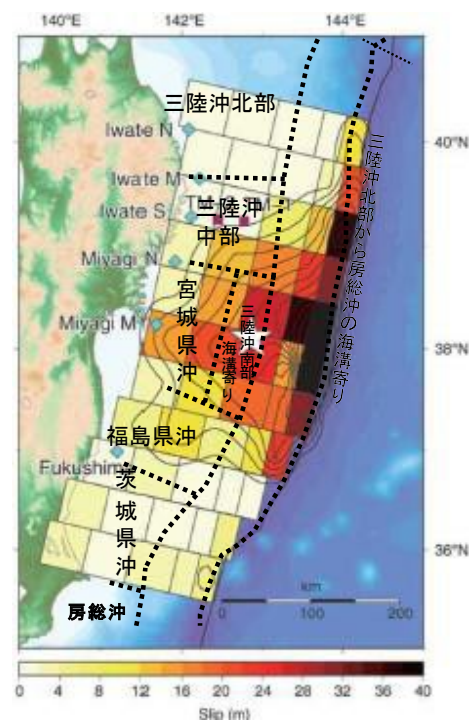
津波インバージョン解析 (Satake et al. (2013)に加筆)
