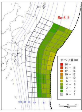
延宝房総沖地震(Mw 8.5)
