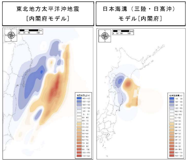
東北地方太平洋沖地震(Mw 9.0) 日本海溝沿い地震(Mw 9.1) (宮城県(2022))
