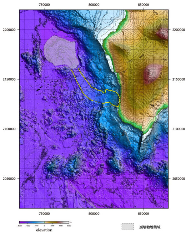
「Alika-2」の海底地すべり判読結果(現況地形)
