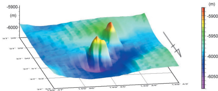
図4 北北東から眺めた2つのプチスポット火山の鳥瞰図。山体の規模は、いずれも長径1 km、比高100~200 m程度である。調査船による音波を用いた海底地形探査でやっと初めてその存在が明らかとなる大きさである。網度程度を示すグリッドは1分がおおよそ1.85 kmに相当。図2の幅幅が約1100 kmであるのに対し、この図の幅幅はたった7.4 kmに過ぎないことに注意。
