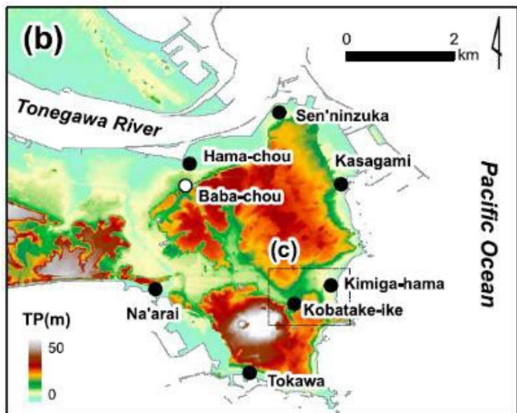
(b)千葉県銚子市付近の標高分布と古文書に基づく1677年の津波の影響範囲 (●:津波被害あり, ○:津波被害なし)
