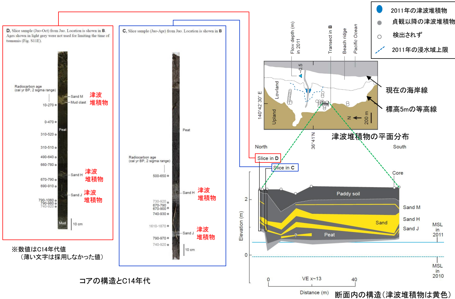
茨城県日立市十王町における津波堆積物調査結果の概要(Sawai et al.(2012)に加筆)
