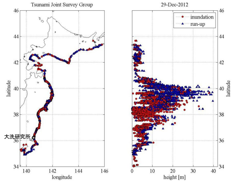
2011年東北地方太平洋沖地震による浸水高及び遡上高分布図 (東北地方太平洋沖地震津波合同調査グループ(2011)に加算)
