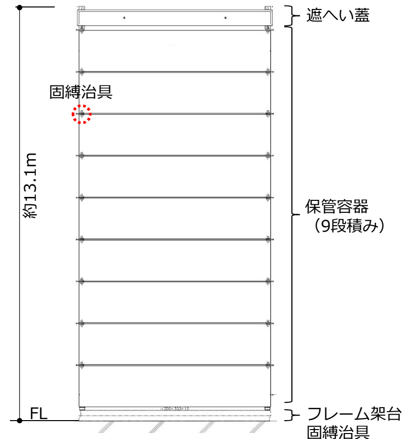
保管容器9段積み（立面図・イメージ）
