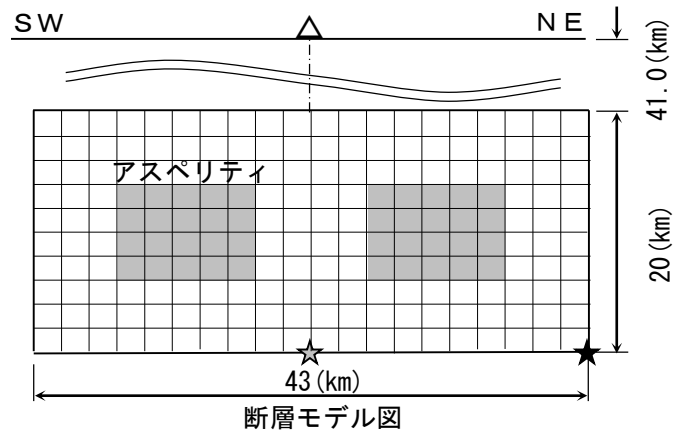
☆☆ : 破壊開始点
