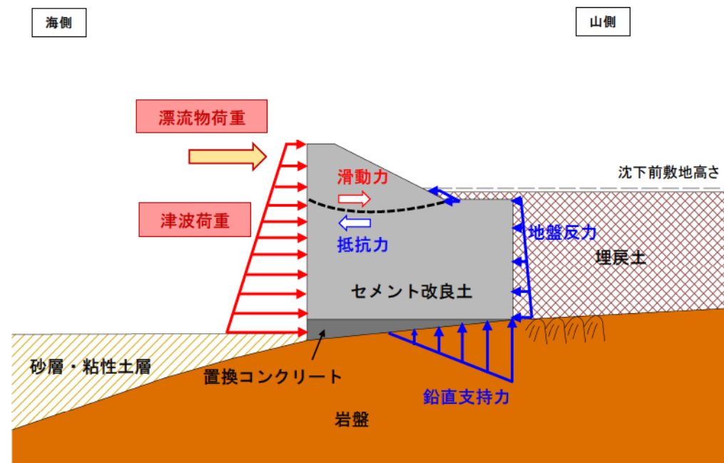
荷重図
