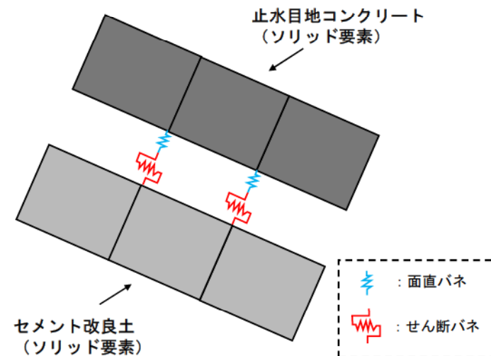
止水目地コンクリートとセメント改良土の境界部のモデル化イメージ
