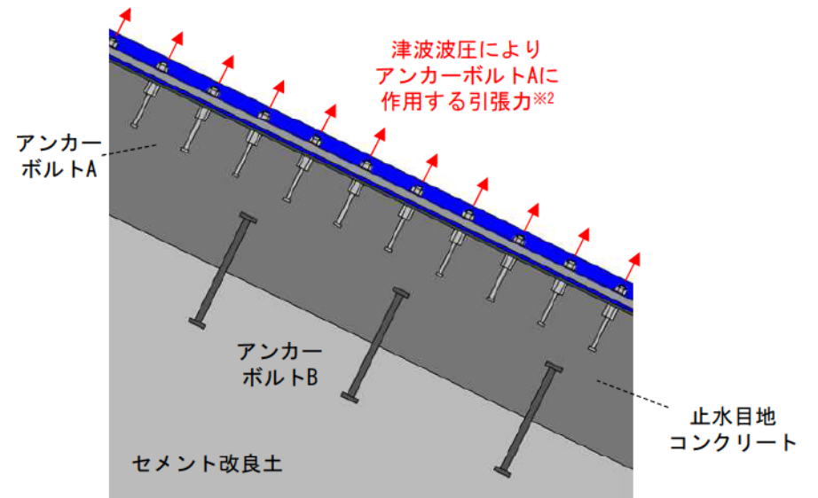
津波時にアンカーボルトBに生じる外力
