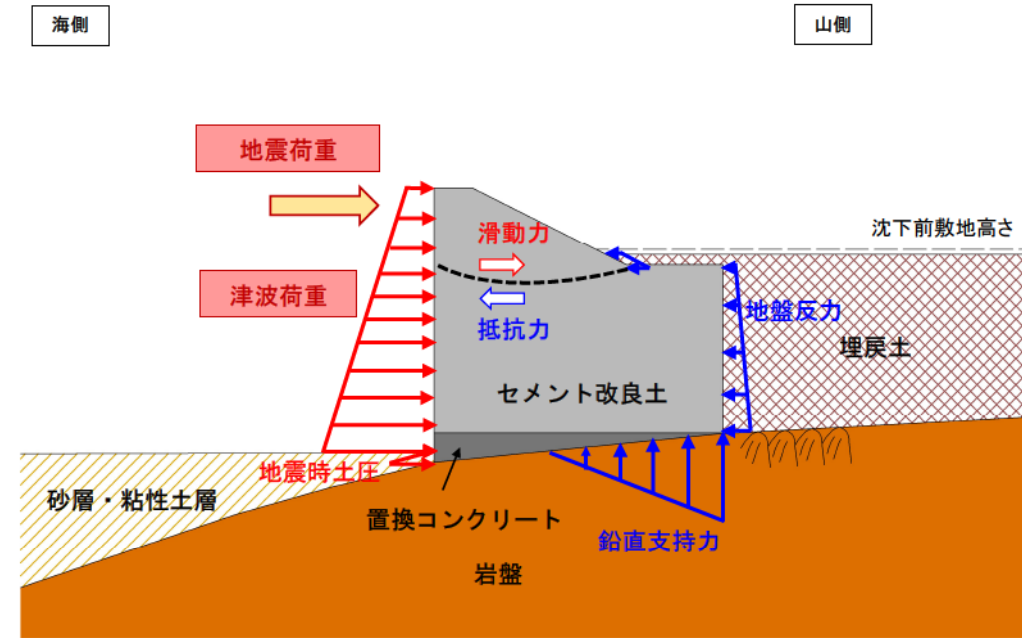
荷重図
