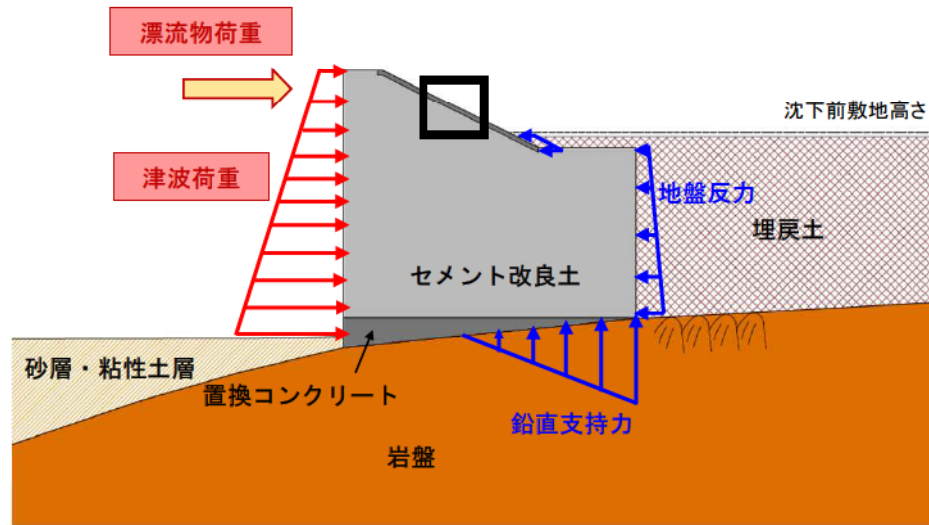
津波時に防潮堤に生じる外力
