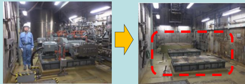
○浜岡 1 号機ほう酸注入系 (原子炉建屋内)
