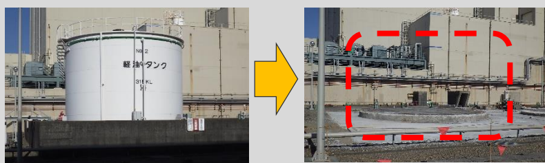
○浜岡2号機軽油タンク解体（屋外）
