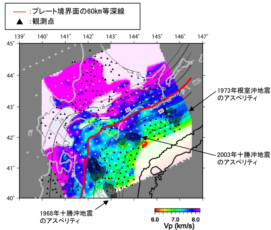
プレート境界面直下5kmにおけるVpの分布とプレート境界地震の破壊域、相似地震の震央の分布との比較 (文部科学省(2008)一部加筆)
