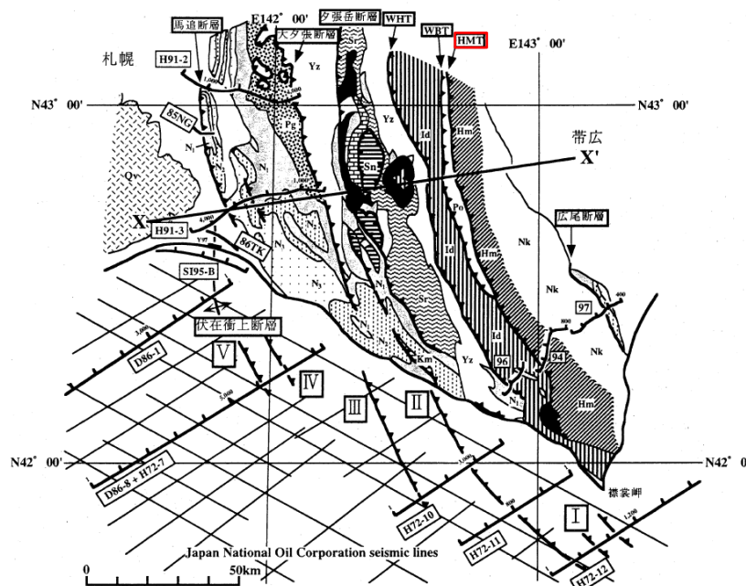
図1 日高衝突帯ならびに前縁褶曲・衝上断層帯の地質概略と主な反射法地震探査測線図。X-X'は図2の断面位置を示す。伊藤ら(1999)を改変。 【地質】主として、地質調査所(1982, 1996)による。Nk: 中の川層群, Hm: 日高変成岩類(主帯), Po: ポロシリ・オフィオライト(西帯), Id: イドンナップ帯, Yz: 蝦夷層群, Sr: 空知層群, Km: 神威古潭変成岩類, Sn: 沙流川層-ニセウ層, Pg: 古第三系, N1~N3: 地質調査所(1982)と同じ。Qv: 第四紀火山岩類。HMT: 日高主衝上断層, WBT: 西縁衝上断層, WHT: 日高西部断層群 【測線】94・96・97: 日高深部構造反射法探査, 85NG・86TK: 浅野ら(1990), Y97: 佐藤ら(1998), その他の測線は石油公団(1973, 1987, 1993, 1996)。
