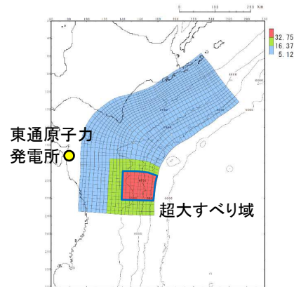
基準断層モデル① (特性化モデル②, 南へ約100km移動)
