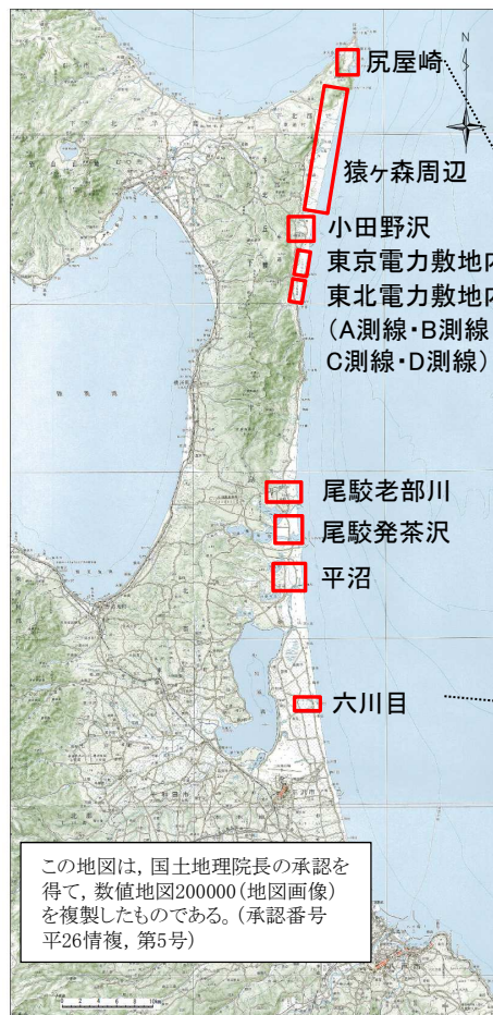
青森県北部太平洋沿岸における津波堆積物の分布(調査位置)
