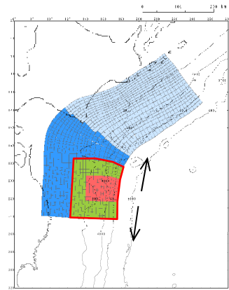
基準断層モデル②(水位下降側)
