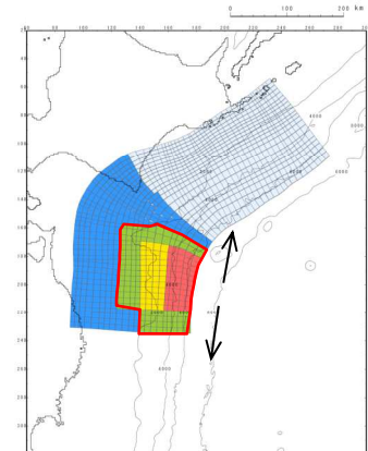
基準断層モデル③(水位下降側)
