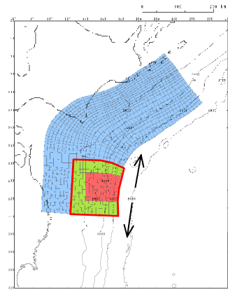
基準断層モデル①(水位上昇側)
