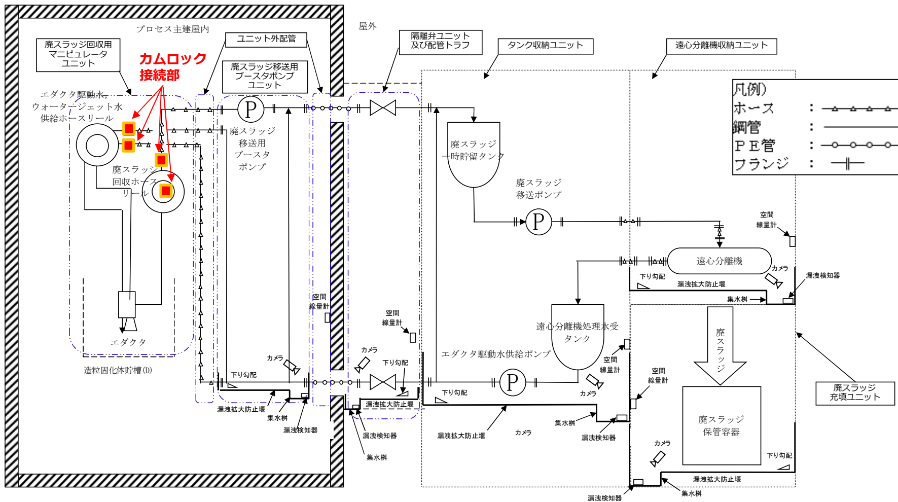
廃スラッジ抜き出し設備
