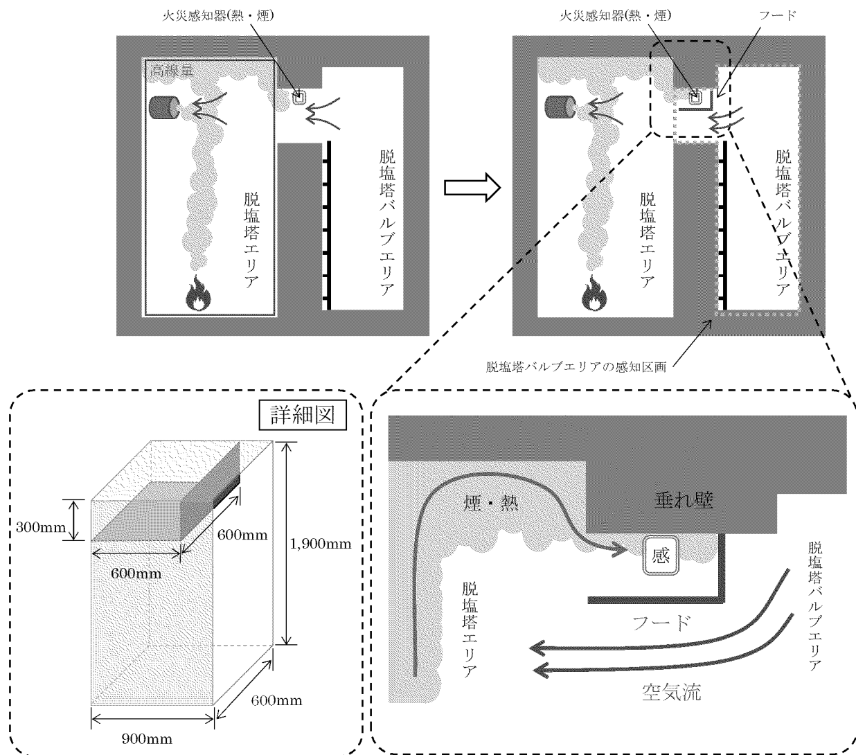
第 7-13 図 脱塩塔エリア開口部におけるフードを用いた火災感知器の設置概要
